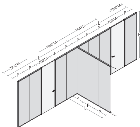
Anta battente / Swing door
