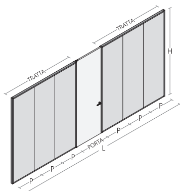
Anta battente / Swing door
