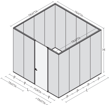
Anta battente / Swing door
