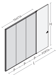
Anta battente / Swing door
