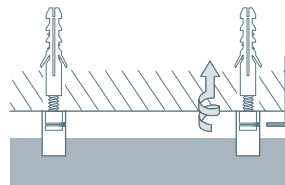
Deckenmontage:
