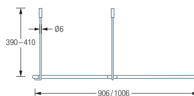
DSFE900K45 / 1000K45 Seitenansicht:
