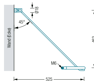
G500VW Seitenansicht:
