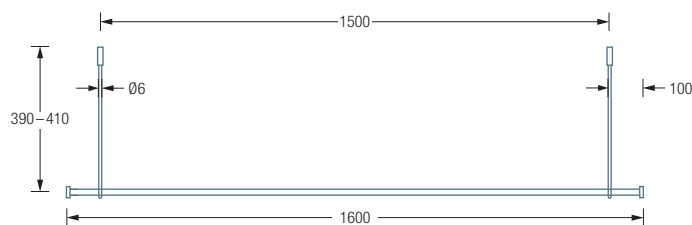
DSN12-1600F Seitenansicht:
