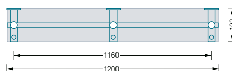
G9-1200G/H Draufsicht:
