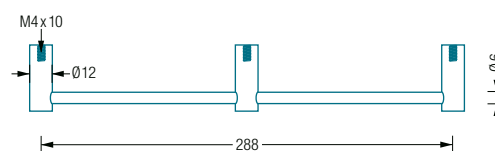
BG6-288E Draufsicht:
