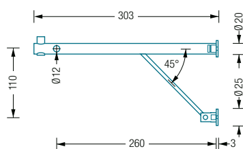
G3-600 / G3-1200 Seitenansicht:
