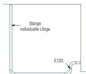
S-förmiger Wandanschluss:
