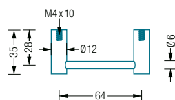
BG6-288E Draufsicht:
