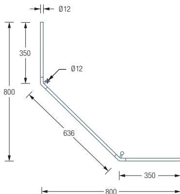
DSFE900 / 1000 Draufsicht:
