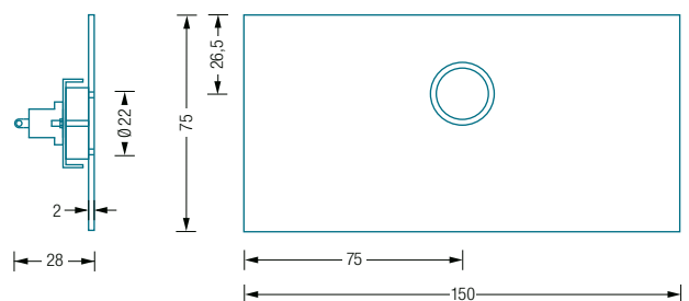
KK75-150M Seitenansicht / Frontansicht:
