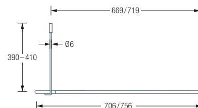
DSU1700-700K45 / 750K45 Seitenansicht:
