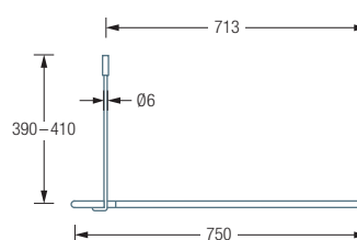
DSE1700-750 Seitenansicht:
