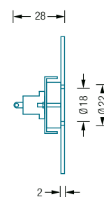
KK75R Seitenansicht:
