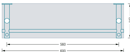
G4-600G/H Draufsicht:
