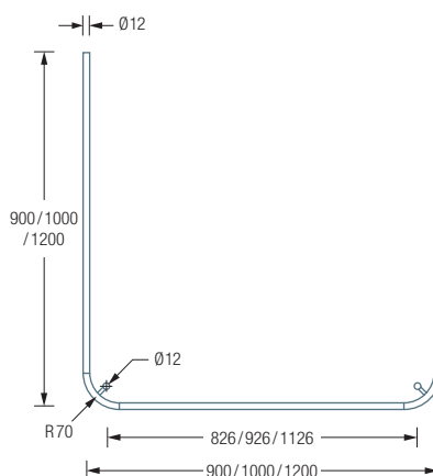
DSU900-900 / 1000-1000 / 1200-1200 Seitenansicht:
