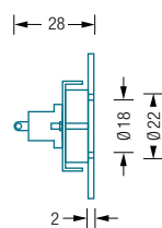
KK50 Seitenansicht:
