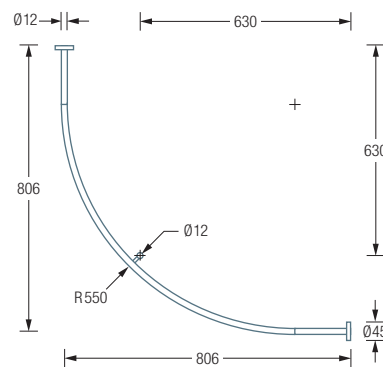
DSB550-800K45 Draufsicht:
