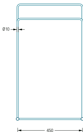
HTB2K Frontansicht:
