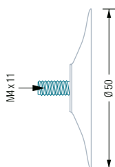
SN50-11 Seitenansicht:
