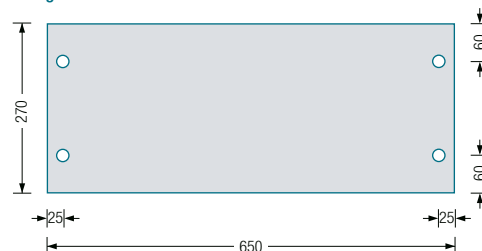
Ablage G3-600G/H Draufsicht:
