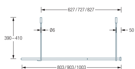
DSB550-800F / 900F / 1000F Seitenansicht:
