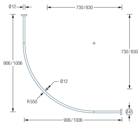
DSB550-900K45 / 1000K45 Draufsicht:
