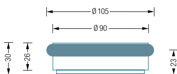
TSB90-30 Seitenansicht:
