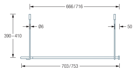
DSU1700-700F / 750F Seitenansicht:
