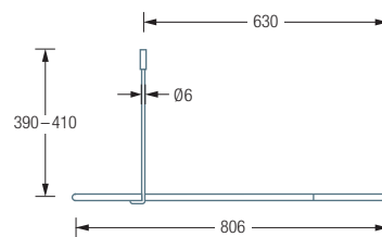
DSB550-800K45 Seitenansicht:
