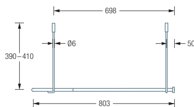
DSB300-800F Seitenansicht:
