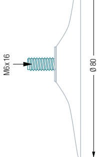
SN80-16/-16S Seitenansicht:
