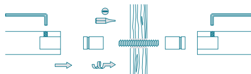
Beidseitige Verschraubung* – Bohrung in Paneel Ø 6/8 mm
