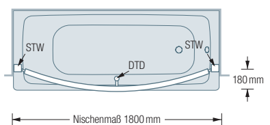
DSGN12 Draufsicht – mit Radius 1800 mm:
