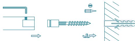
Wandverschraubung – Bohrung in Wand Ø 6/8 mm
