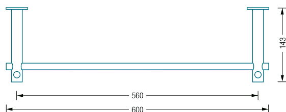
G4-600 Draufsicht:
