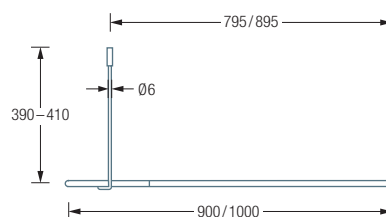
DSB300-900 / 1000 Seitenansicht:
