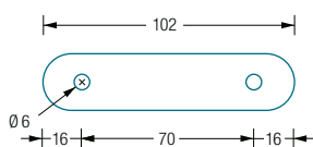
ROV23-B6 Draufsicht:
