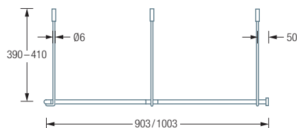
DSFE900F / 1000F Seitenansicht:
