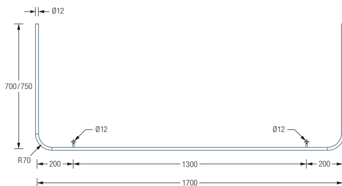
DSU1700-700D / 750D Draufsicht:
