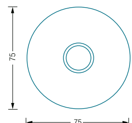
KK75R Frontansicht:
