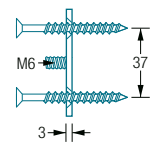
R55VN Seitenansicht:
