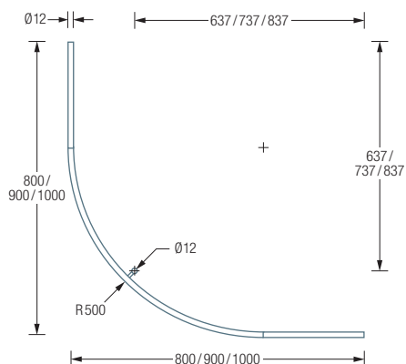
DSB500-800 / 900 / 1000 Draufsicht:
