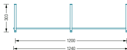
G3-1200 Draufsicht:
