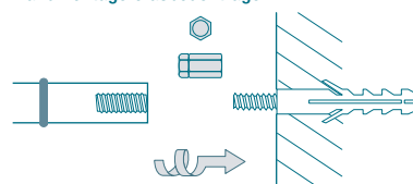
Wandmontage Glasbodenträger:
