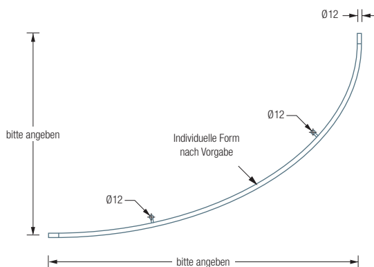
DSGE12 Draufsicht:
