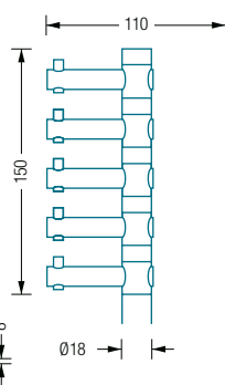
360° Drehhaken:
