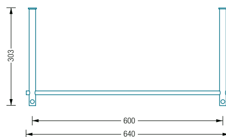
G3-600 Draufsicht:
