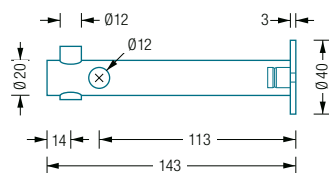
G4-600 / G4-1200 Seitenansicht:
