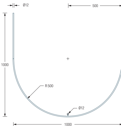
DR500HD1000 Seitenansicht:
