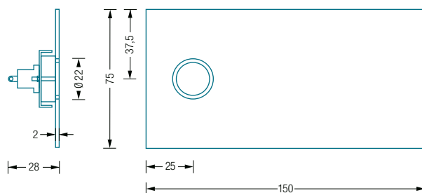
KK75-150S Seitenansicht / Frontansicht:
