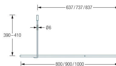
DSB500-800 / 900 / 1000 Seitenansicht:
