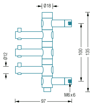
GH3 Seitenansicht:
