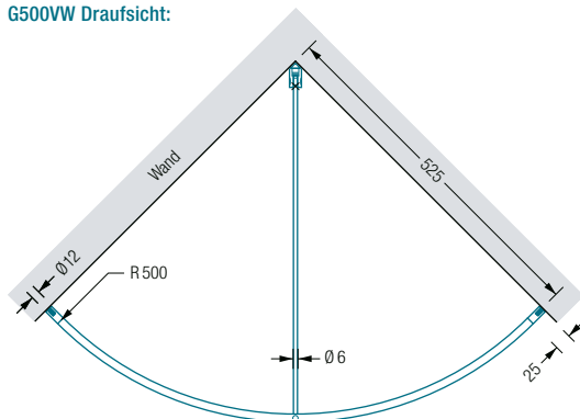
G500VW Draufsicht:
