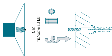
TSB80-13 Wandmontage über M10 Adapter auf M6 Stockschraube:
