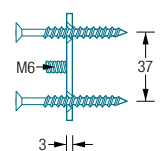
R55S Seitenansicht:
