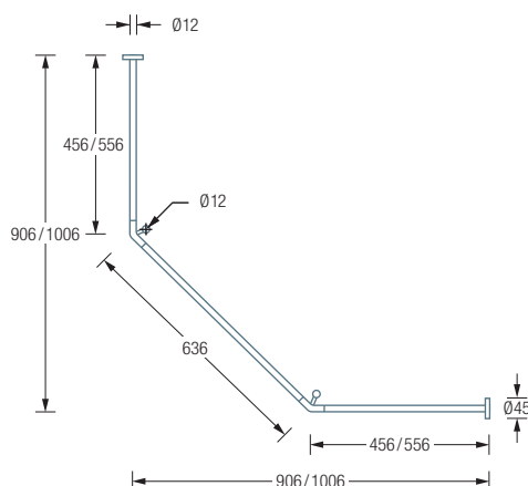
DSFE900K45 / 1000K45 Draufsicht:
