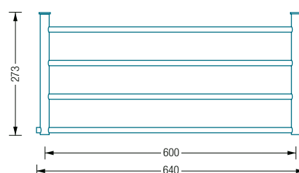
G5-600 Draufsicht:
