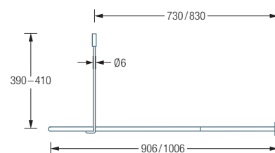
DSB550-900K45 / 1000K45 Seitenansicht:
