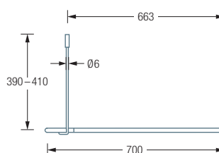
DSE1700-700 Seitenansicht:
