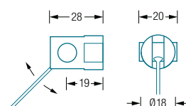
Winkelflexible Wandbefestigung:
