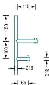
GSTS2S-B Detailansicht:
