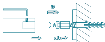
Wandverschraubung – Bohrung in Wand Ø 8 mm
