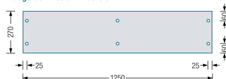
Ablage G5-1200G/H Draufsicht:
