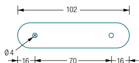
ROV23-B4 Draufsicht:
