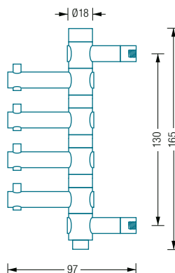
GH4 Seitenansicht:
