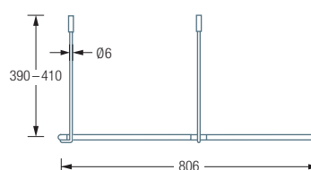
DSFE800K45 Seitenansicht:
