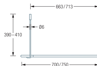
DSU1700-700D / 750D Seitenansicht:
