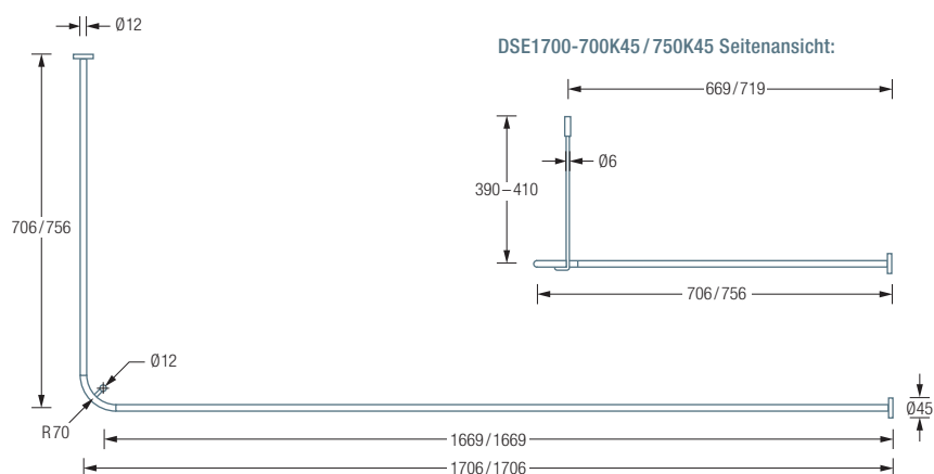
DSE1700-700K45 / 750K45 Draufsicht:
