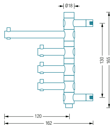
GH4-2 Seitenansicht:
