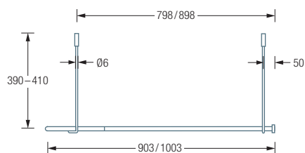
DSB300-900F / 1000F Seitenansicht:
