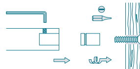
Rückseitige Verschraubung* – Bohrung in Paneel Ø 6/8 mm
