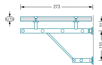
G8-600/1200G/H Seitenansicht:
