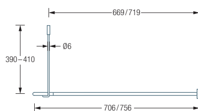
DSE1700-700K45 / 750K45 Seitenansicht:
