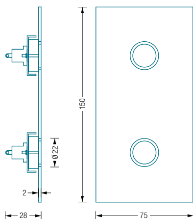
KK150-75 Seitenansicht / Frontansicht:
