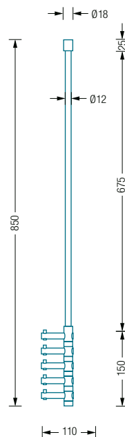
T5 Seitenansicht:
