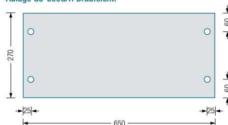
Ablage G5-600G/H Draufsicht:
