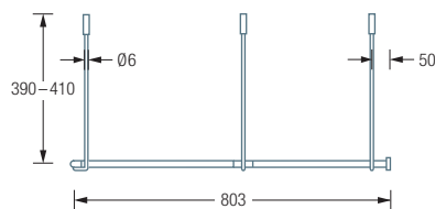
DSFE800F Seitenansicht:
