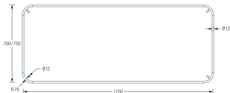
DSRE1700-700 / 750 Draufsicht:
