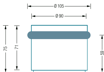
TSB90-75 Seitenansicht:
