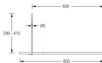
DSB300-800 Seitenansicht:
