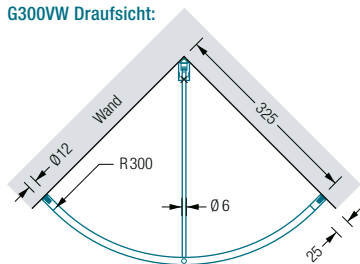
G300VW Draufsicht:
