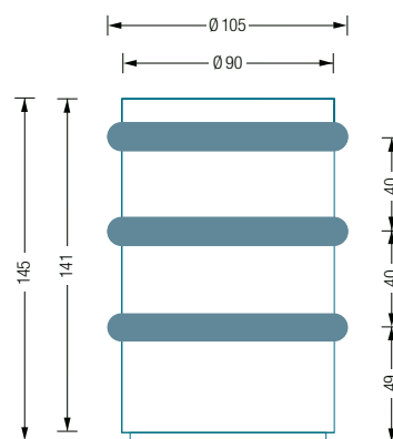
TSB90-145 Seitenansicht:
