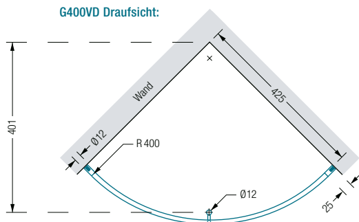
G400VD Draufsicht:
