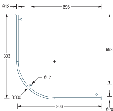
DSB300-900F / 1000F Draufsicht:
