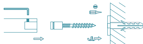
Wandverschraubung mit Rosette – Bohrung in Wand Ø 6/8 mm
