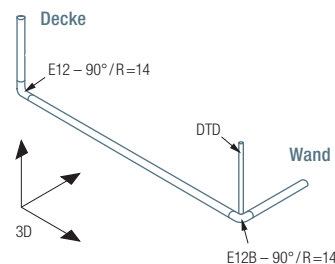
U-Form, 90° verdreht:
