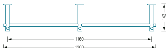
G4-1200 Draufsicht:
