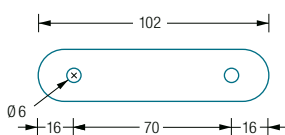
ROV23-B6 Draufsicht:
