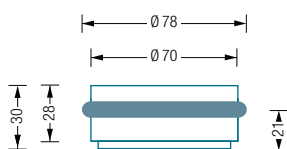
TSB70-30 Seitenansicht:
