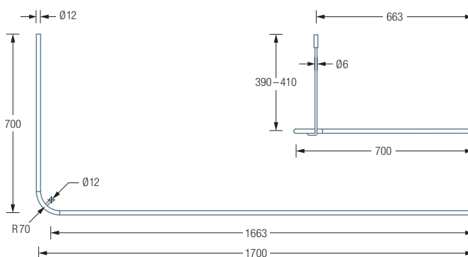
DSE1700-700 Draufsicht:
