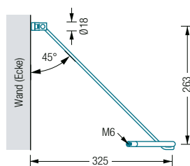
G300VW Seitenansicht:
