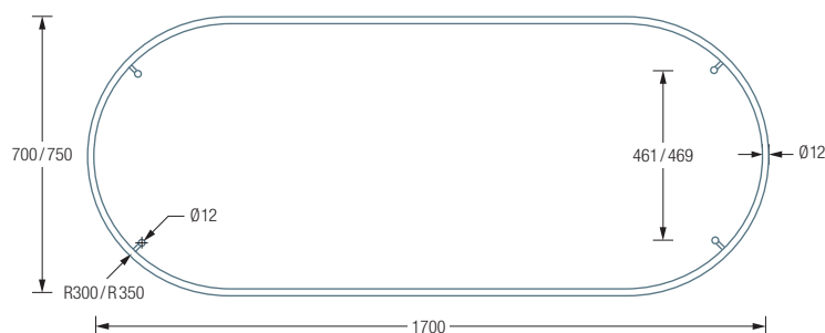
DS01700-700 / 750 Draufsicht:
