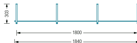
G3-1800 Draufsicht:
