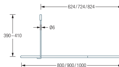
DSB550-800 / 900 / 1000 Seitenansicht:
