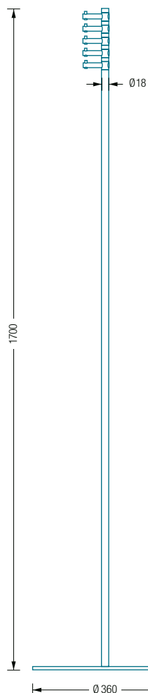
360° Drehhaken:
