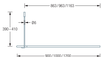
DSU900-900 / 1000-1000 / 1200-1200 Seitenansicht:
