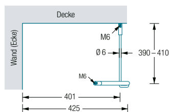
G400VD Seitenansicht:
