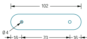
ROV23-B4 Draufsicht:
