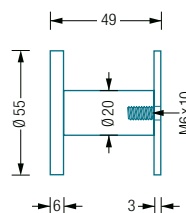
HA3-R55S55-B Seitenansicht:
