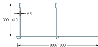
DSFE900 / 1000 Seitenansicht:
