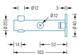
G9-600 / G9-1200 Seitenansicht:
