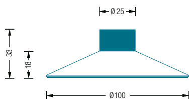
TSB100-18 Seitenansicht:
