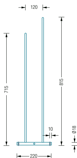
HTB2K Seitenansicht:
