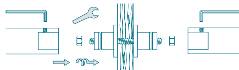
Beidseitige Verschraubung* – Bohrung durch Paneel Ø 6 mm
