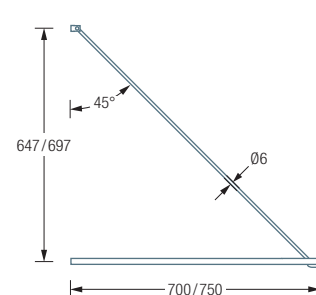
DSU1700-700W / 750W Seitenansicht:
