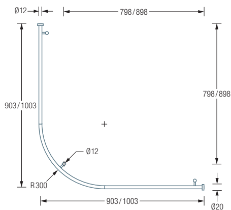
DSB300-900F / 1000F Draufsicht:
