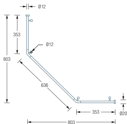
DSFE800F Draufsicht:
