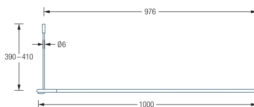
DR500HD1000 Seitenansicht:
