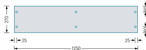
Ablage G3-1200G/H Draufsicht:
