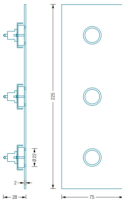
KK225-75 Seitenansicht / Frontansicht:
