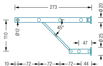
G8-600 / G8-1200 Seitenansicht:
