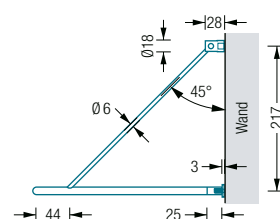
GU1-1600 Seitenansicht:
