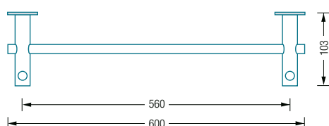
G9-600 Draufsicht:
