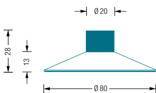
TSB80-13 Seitenansicht:
