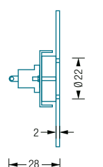
KK75S Seitenansicht:
