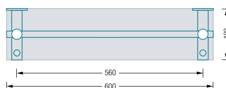
G9-600G/H Draufsicht:
