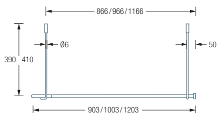
DSE900F / 1000F / 1200F Seitenansicht:
