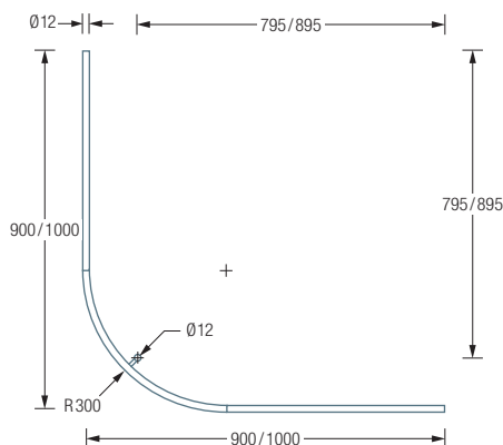
DSB300-900 / 1000 Draufsicht:
