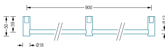
BG12-900E Draufsicht:
