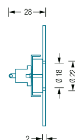
KK75R Seitenansicht:
