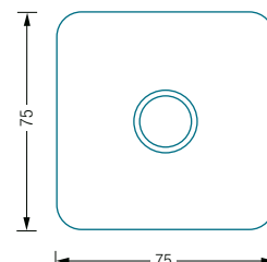
KK75S Frontansicht:
