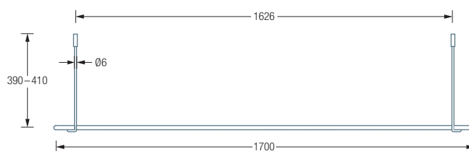
DSRE1700-700 / 750 Seitenansicht:
