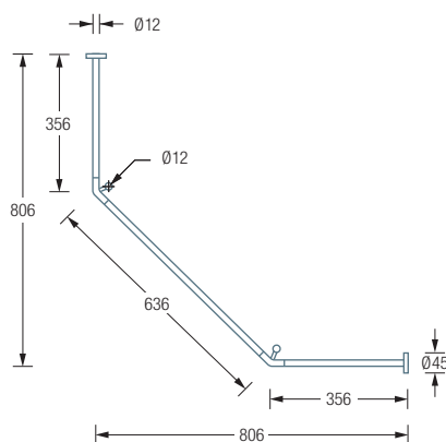
DSFE900K45 / 1000K45 Draufsicht:
