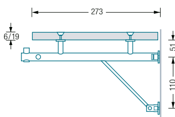
G3-600/1200G/H Seitenansicht:
