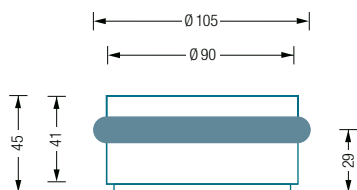
TSB90-45 Seitenansicht:
