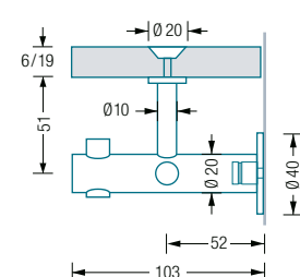
G9-600/1200G/H Seitenansicht:
