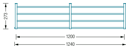
G8-1200 Draufsicht:
