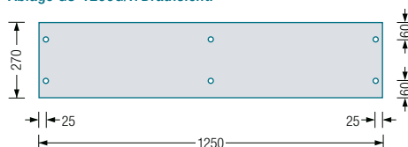
Ablage G8-1200G/H Draufsicht:
