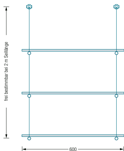
RST260-3 Frontansicht:
