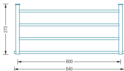
G8-600 Draufsicht:
