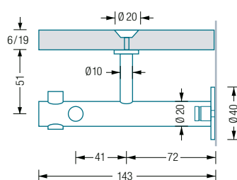
G4-600/1200G/H Seitenansicht:
