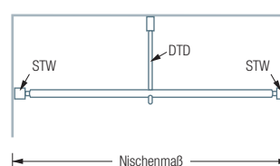
DSGN12 Frontansicht:
