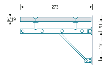
G5-600/1200-Glas/H Seitenansicht:
