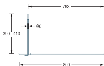
DSU800-800 Seitenansicht:
