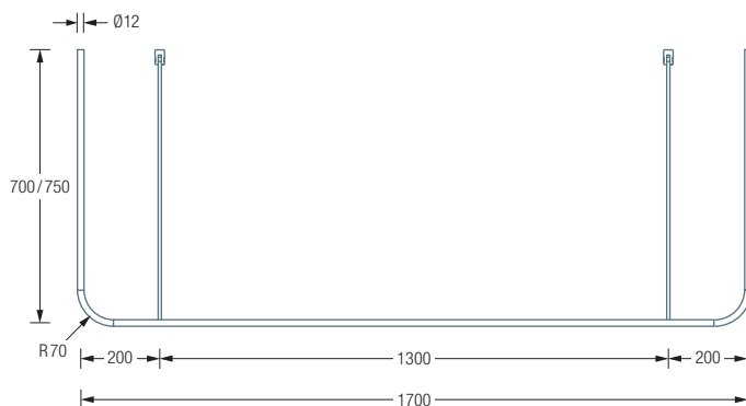
DSU1700-700W / 750W Draufsicht:
