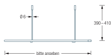
DSGE12 Seitenansicht:
