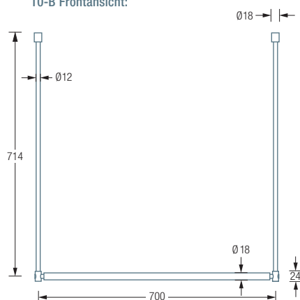
T0-B Frontansicht:
