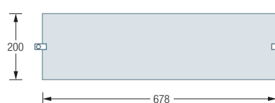
TOG-B Glasablage Draufsicht:
