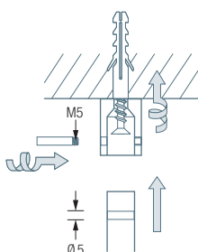
Deckenmontage mit Befestigungselement DL12:
