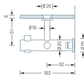
G9-500G-B / 600G-B Seitenansicht:
