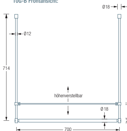
TOG-B Frontansicht:
