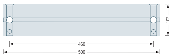
G9-500G-B Draufsicht:
