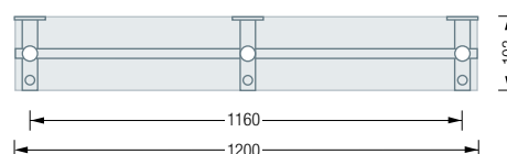
G9-1200G/H Draufsicht:
