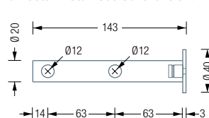
G7-600/-1200/-1800 Seitenansicht:
