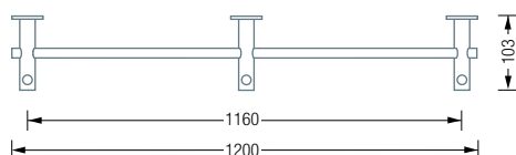
G9-1200 Draufsicht:
