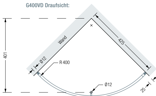
G400VD Draufsicht:
