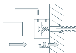
Wandmontage mit Wandlager WL18:
