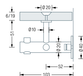
G9-600/1200G/H Seitenansicht:
