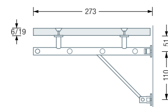
G5-600/1200G/H Seitenansicht:
