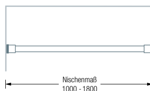
TKS20-2 Frontansicht:
