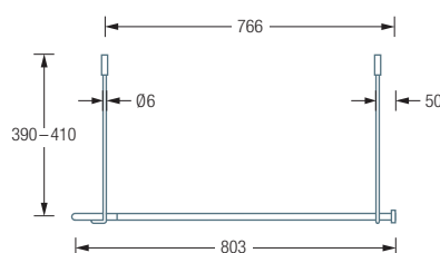
DSE800F Seitenansicht:
