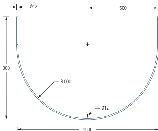
DR500HD800 Seitenansicht:
