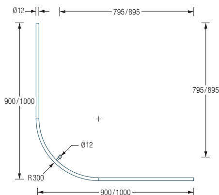
DSB300-900 / 1000 Draufsicht:
