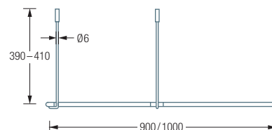
DSFE900 / 1000 Seitenansicht:
