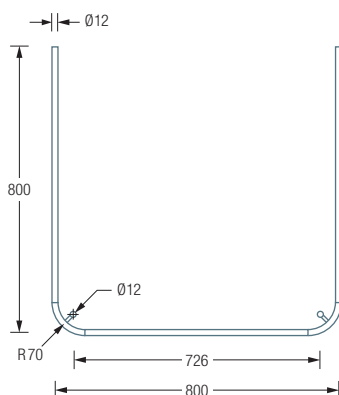
DSU800-800 Seitenansicht:
