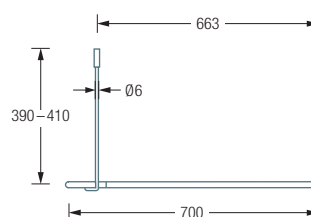
DSE1700-700 Seitenansicht:
