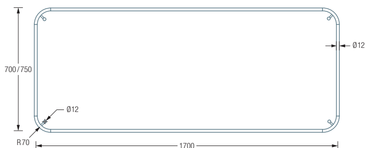
DSRE1700-700 / 750 Draufsicht:
