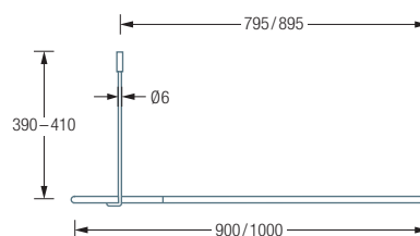
DSB300-900 / 1000 Seitenansicht:
