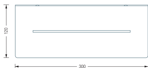
DA300 Rückansicht:
