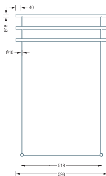
HTB3 Frontansicht:
