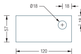
BA200 / 290 Seitenansicht:
