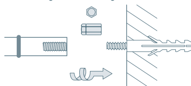
Wandmontage Glasbodenträger:
