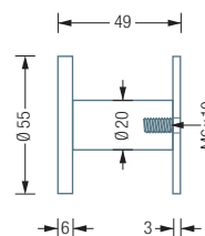
HA3-R55S55-B Seitenansicht:
