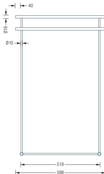
HTB2 Frontansicht:
