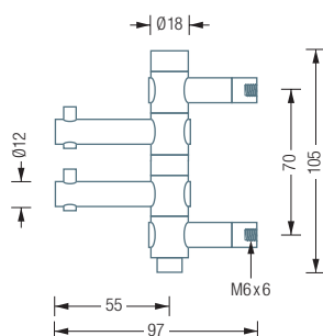
GH2-B Seitenansicht:
