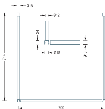
T0-B Frontansicht:
