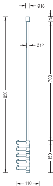
T5-B Seitenansicht:
