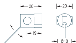
Winkelflexible Wandbefestigung:
