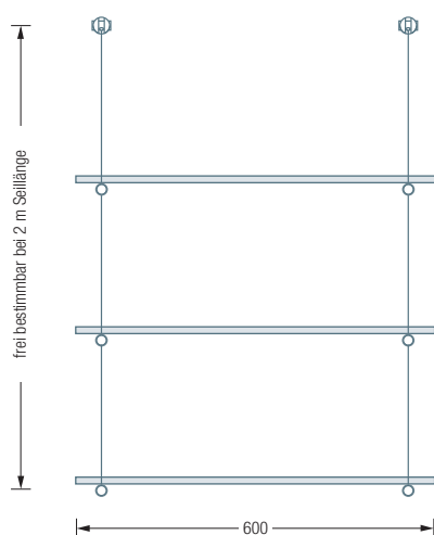
RST260-3-B Frontansicht:
