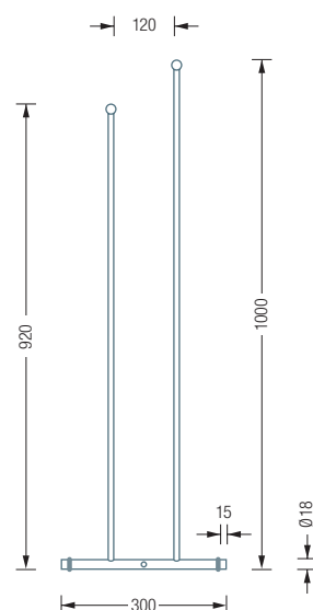
HTB2 Seitenansicht:
