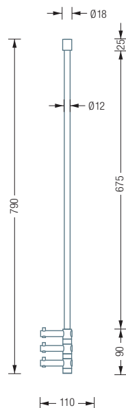
T3-B Seitenansicht:
