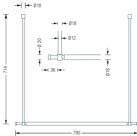
T0S-B Frontansicht:
