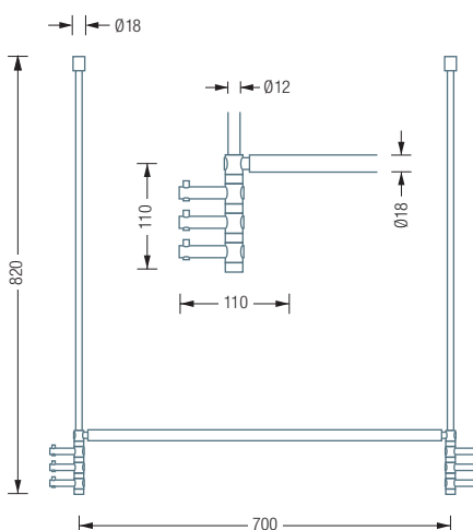
T3D-B Frontansicht:
