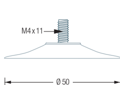
SN50-11 Seitenansicht:
