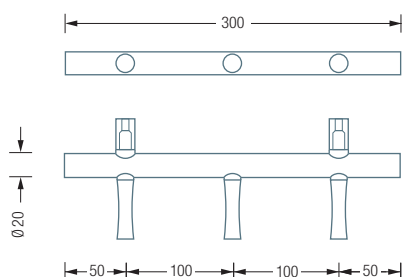
HLS3F-B – HAKENLEISTE FLOW
