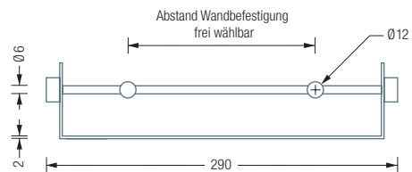
BA290 Frontansicht:
