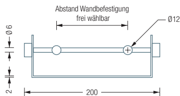
BA200 Frontansicht:
