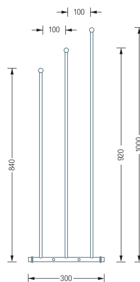
HTB3 Seitenansicht:
