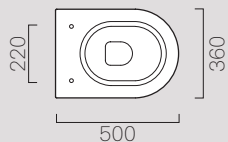
Curva tecnica Technical curve
