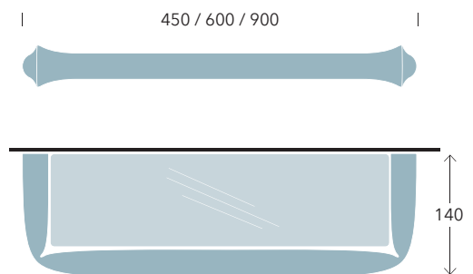
art. FL45M / FL60M / FL90M mensola con piano in cristallo crystal shelf tablette en verre Ablage mit Fläche aus Kristallglas dim. 45 / 60 / 90 x 14 cm
