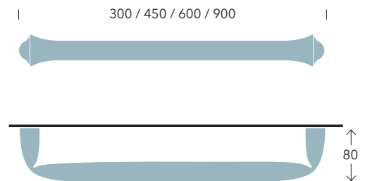
art. FL45M / FL60M / FL90M mensola con piano in cristallo crystal shelf tablette en verre Ablage mit Fläche aus Kristallglas dim. 45 / 60 / 90 x 14 cm
