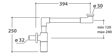
Space-saving siphon 1"1/4, weight: 1,16 kg Platzsparender Siphon 1"1/4, Gewicht 1,16 kg
