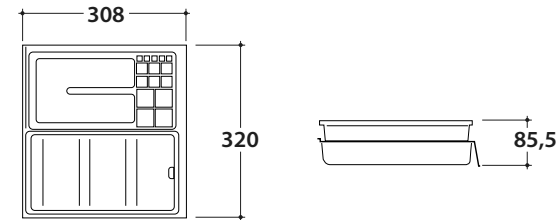
Large container 32x31 h9 cm Großer Behälter 32x31 h9 cm
