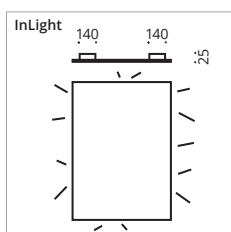
Lichtprofil eingerückt
