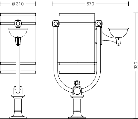
Melia 2274.002 M • Ghisa e acciaio zincato • Capacità 37l
