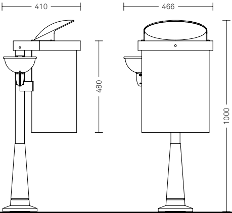
Gilia – con copertura 2273.002 M • Ghisa, alluminio, acciaio zincato • Capacità 33,5l
