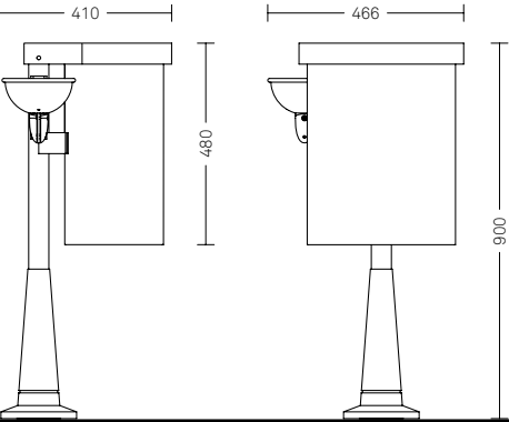
Gilia 2273.003 M • Ghisa, alluminio, acciaio zincato • Capacità 33,5l
