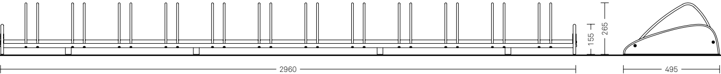
Portabici 2285.001 T • Ghisa e acciaio zincato
