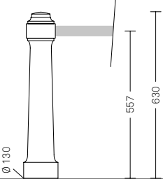
Nyssa – colonna 2989.000 M
