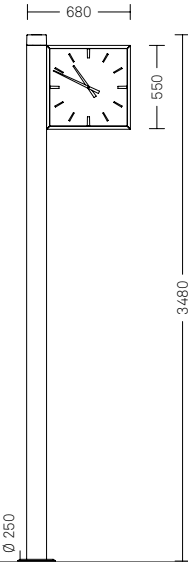
Lilium 2209.000 F • Alluminio • Cassa in alluminio a due quadranti color argento
