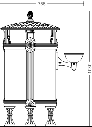
Layia 2270.000.002 M • Alluminio e acciaio zincato • Capacità 50l
