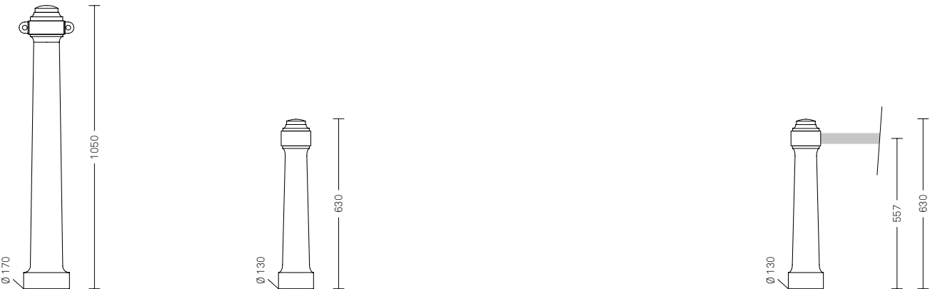
Dissuasore 2985.000 M 2985.001 R • Ghisa sferoidale
