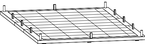
Basamento livellante completo di pedana in legno o pavimento flottante in gres porcellanato (in mancanza di una fondazione a platea o a cordolo è possibile installare il chiosco utilizzando questa piattaforma)
