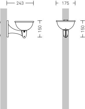
Melia – per tubi 2800.001 V 2800.002 V 2800.003 V Posacenere con placca per tubi da: Ø 33mm (2800.001) Ø 48mm (2800.002) Ø 60mm (2800.003) • Ghisa
