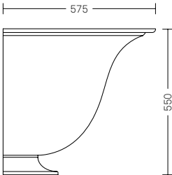
Salix – a parete 2204.001 T • Ghisa • Capacità 100l
