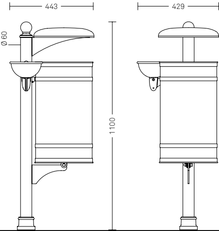
Melia – con copertura 2275.001.002 C1 M 2275.101.002 C2 M C1 cesto singolo C2 cesto doppio • Ghisa e acciaio zincato • Capacità 37l (cesto singolo) e 74l (cesto doppio)
