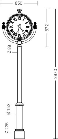
Melia 2211.000.003 M • Ghisa, acciaio e alluminio • Cassa in fusione di alluminio con due quadranti color bianco
