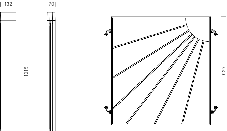
Lilium – colonna 2968.000 M
