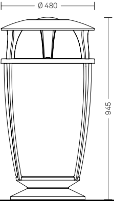
Idesia 2277.002 T • Alluminio e acciaio zincato • Capacità 75l
