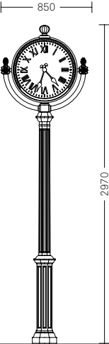
Scilla 2211.000 M • Ghisa, acciaio e alluminio • Cassa in fusione di alluminio a due quadranti color bianco
