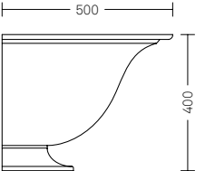
Salix – a parete 2203.001 T • Ghisa • Capacità 57l
