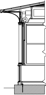
Codice XXXX.XXX.310 Chiosco davanzale basso
