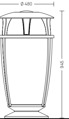
Cestino con posacenere 2277.002 T • Alluminio e acciaio zincato • Capacità 75l
