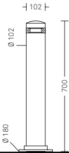
Dissuasore 2975.000 M 2975.001 R • Ghisa sferoidale
