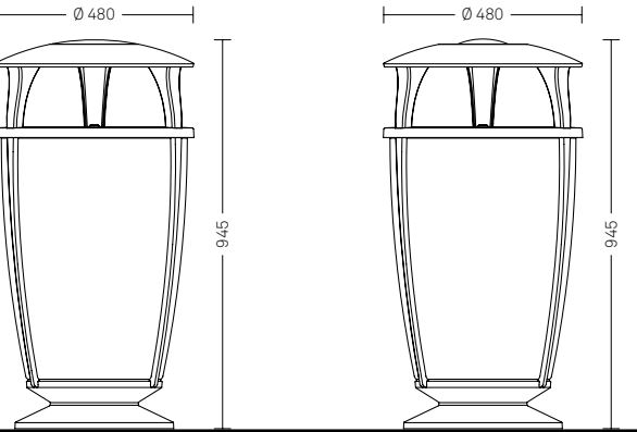
Cestino 2277.001 T • Alluminio e acciaio zincato • Capacità 75l
