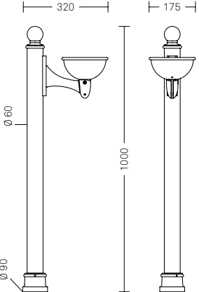
Melia – a colonna 2800.004 M • Ghisa e acciaio zincato
