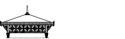
Codice XXXX.005.XXX Tetto a falde con sporgenza ridotta (disponibile solo per i chioschi con codice pianta 3004, 3005, 3006)
