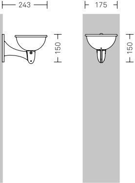
Melia – a parete 2800.000 Posacenere oscillante per svuotare la cenere • Ghisa
