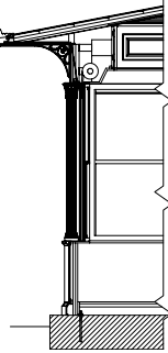
Codice XXXX.XXX.300 Chiosco davanzale basso
