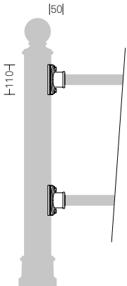
Collare 9502.905
