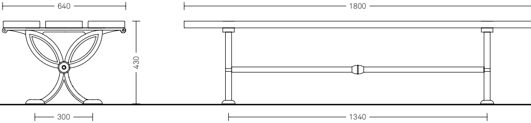
Panchina 2171.002.018 M • Seduta in legno Iroko marrone • Piede in ghisa
