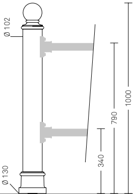
Melia – colonna 2971.050 M
