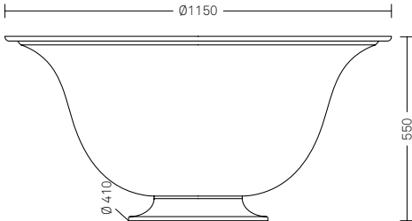
Salix 2204.000 T • Ghisa • Capacità 200l
