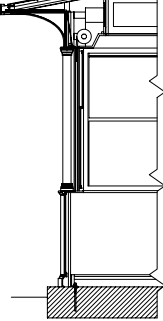
Codice XXXX.XXX.610 Chiosco altezza maggiorata
