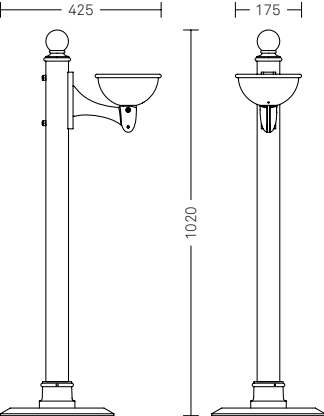
Melia – a piantana 2800.004.001 P • Ghisa e acciaio zincato
