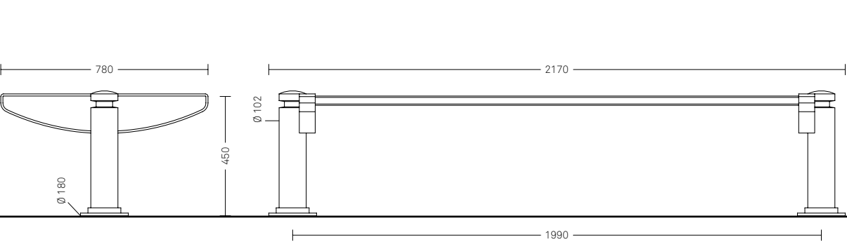
Panchina 2194.002.010 M • Seduta in legno Iroko marrone • Piede in ghisa
