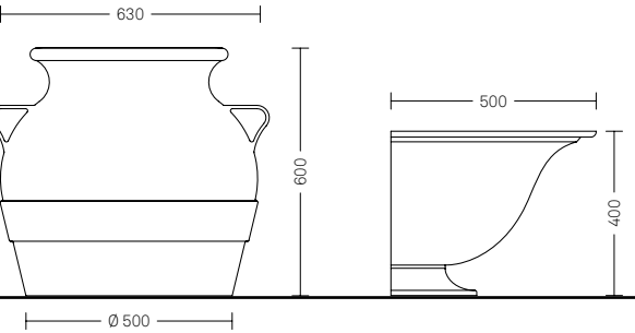
Layia 2212.000.001 T • Ghisa • Capacità 125l
