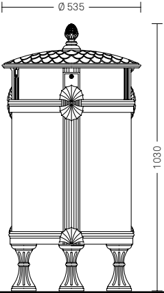
Layia 2270.000 M
