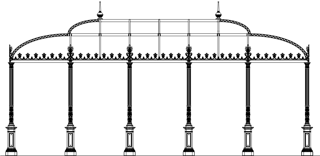
Codice XXXX.100 Altezza maggiorata e interasse colonna di 2m
