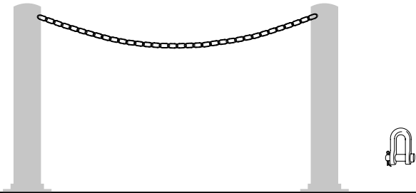
Catena 9525.411.002 Accessorio per dissuasore al metro lineare • Acciaio zincato a caldo e verniciato • Ø 32mm
