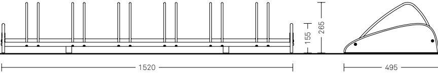
Portabici 2285.000 T • Ghisa e acciaio zincato
