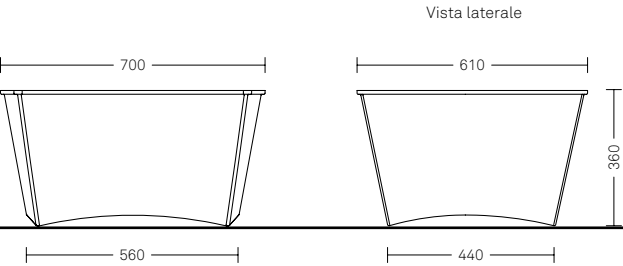
Idesia – componibile 2206.000 T • Ghisa • Capacità 90l
