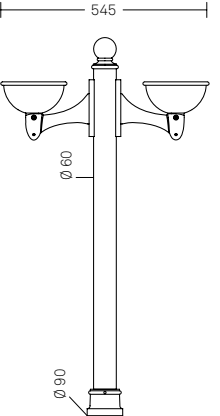
Melia – a colonna 2800.005 M • Ghisa e acciaio zincato
