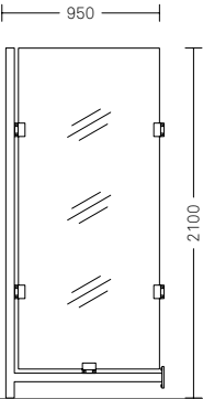
Tamponamento laterale 0002.403.001
