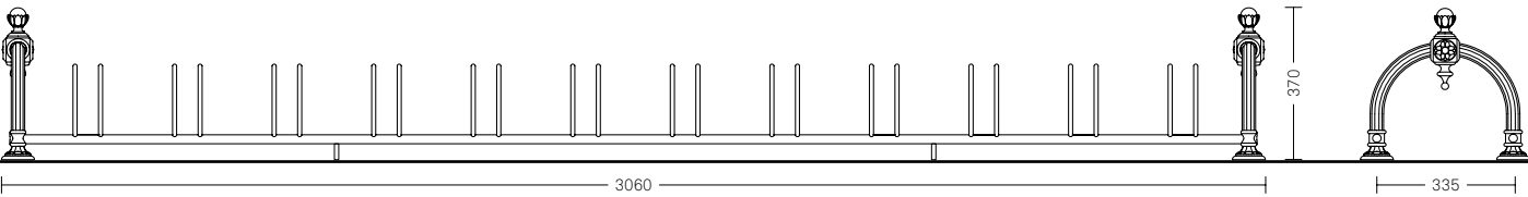
Portabici 2282.001 M
