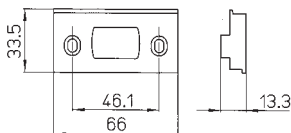
PI286 Controbordo in nylon nero per profilati in alluminio
