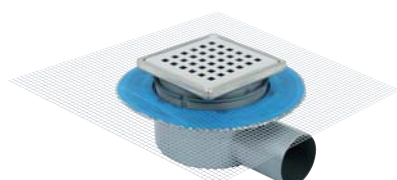
SCARICO ORIZZONTALE ORIENTABILE A 360°
