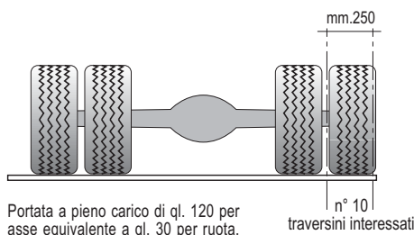
CARICO DISTRIBUITO
