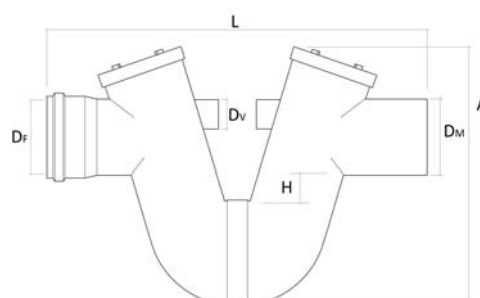
SMS140 - SMS160 - SMS200 SMG160 - SMG200
