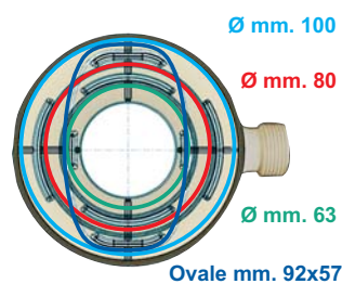
INNESTO DEL TUBO PLUVIALE INFERIORE
