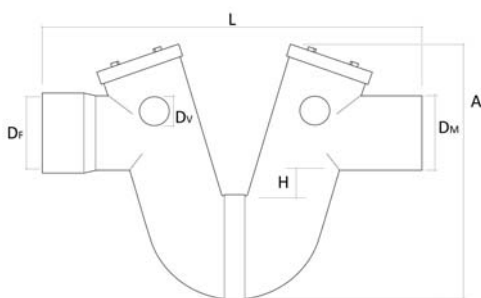
SMS100 - SMS125 SMG100 - SMG125
