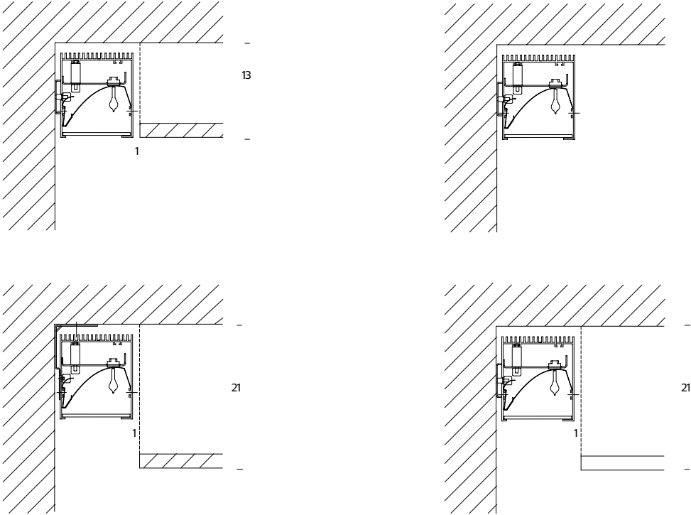
Schema di montaggio consigliato / Recommended assembly diagram / Schéma de montage conseillé / Empfohlene aufbauschemen / Esquema de montaje aconsejado
