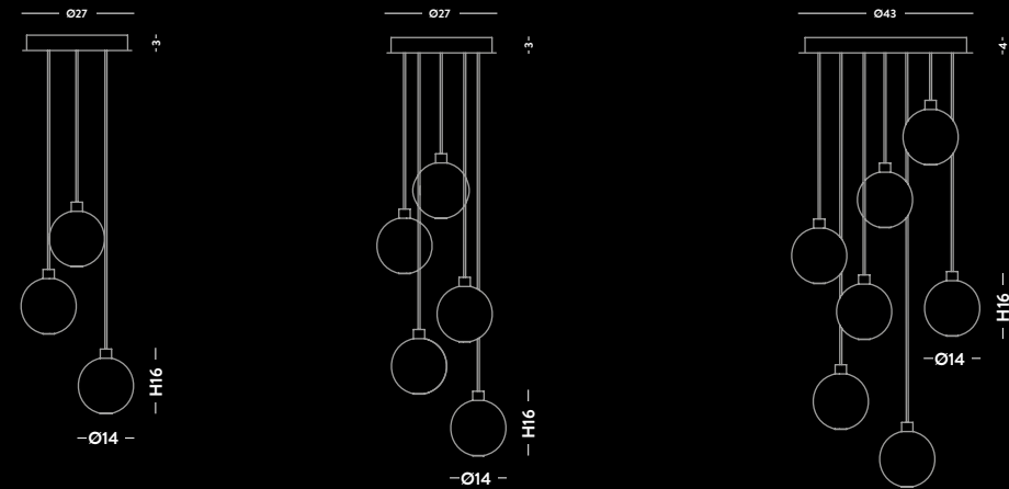
1299.3L Plafoniera / Ceiling lamp vetro/glass Ø14 cm - cavo/cable 150 cm 3 G9 x max 33W 230V CE IP20 1299.5L Plafoniera / Ceiling lamp vetro/glass Ø14 cm - cavo/cable 150 cm 5 G9 x max 33W 230V CE IP20 1299.7L Plafoniera / Ceiling lamp vetro/glass Ø14 cm - cavo/cable 150 cm 7 G9 x max 33W 230V CE IP20
