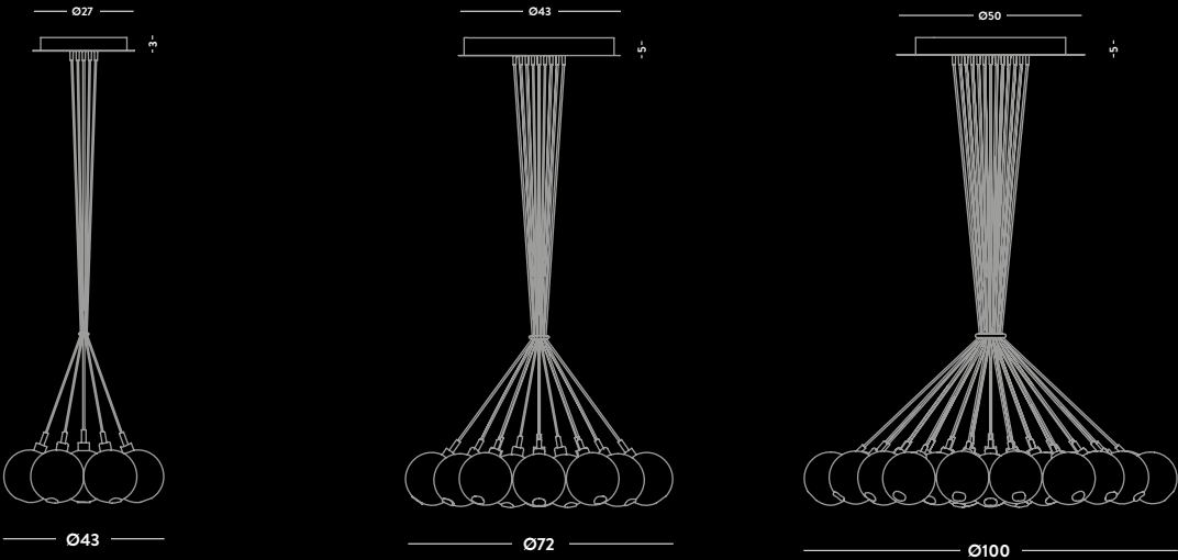
1292.7L Plafoniera / Ceiling lamp vetro/glass Ø14 cm - cavo/cable 150 cm 7 G9 x max 33W 230V CE IP20 1292.19L Plafoniera / Ceiling lamp vetro/glass Ø14 cm - cavo/cable 250 cm 19 G9 x max 33W 230V CE IP20 1292.37L Plafoniera / Ceiling lamp vetro/glass Ø14 cm - cavo/cable 250 cm 37 G9 x max 33W 230V CE IP20
