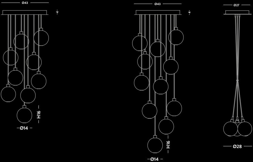
1299.9L Plafoniera / Ceiling lamp vetro/glass Ø14 cm - cavo/cable 150 cm 9 G9 x max 33W 230V CE IP20 1299.11L Plafoniera / Ceiling lamp vetro/glass Ø14 cm - cavo/cable 150 cm 11 G9 x max 33W 230V CE IP20 1292.3L Plafoniera / Ceiling lamp vetro/glass Ø14 cm - cavo/cable 150 cm 3 G9 x max 33W 230V CE IP20
