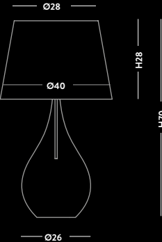
LUGIG1250 Lampada da tavolo / Table lamp vetro/glass Ø26 cm - H70 cm 1 E27 x max 60W 220-240V CE IP20 1m
