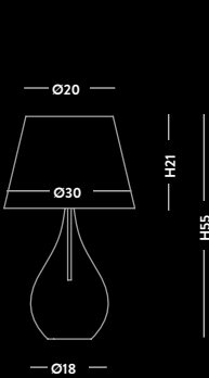
LU1250 Lampada da tavolo / Table lamp vetro/glass Ø18 cm - H55 cm 1 E14 x max 40W 220-240V CE IP20 1m
