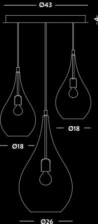
1259MX.3L Plafoniera / Ceiling lamp vetro/glass Ø18/26 cm - cavo/cable 150 cm 2 E14 x max 40W 1 E27 x max 70W 220-240V CE IP20 1m
