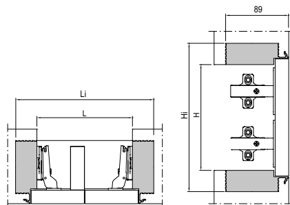
Telaio 4 lati Frame on 4 sides
