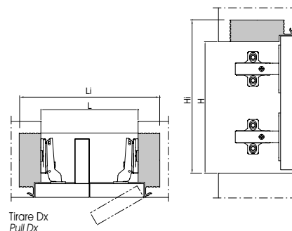
Telaio 3 lati (per altezze 2100 e 2400 mm) Frame on 3 sides (for heights 2100 and 2400 mm)
