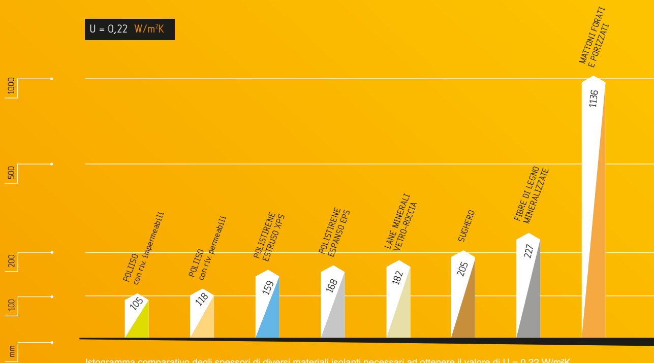
Istogramma comparativo degli spessori di diversi materiali isolanti necessari ad ottenere il valore di U = 0,22 \text{ W/m}^2\text{K}
