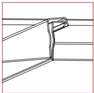
DETTAGLIO AGGANCIO DELLA DOGA INSTALLATION DETAIL
