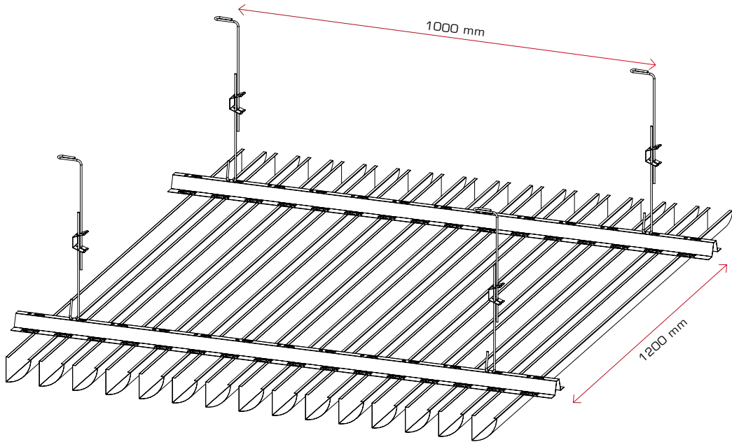
Le doghe STV possono essere installate bidirezionalmente. STV staves can be double face.
