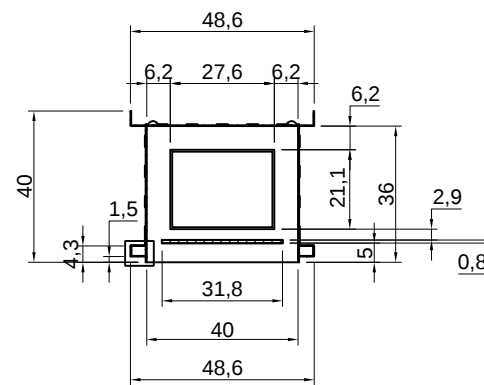
SEZIONE B-B
