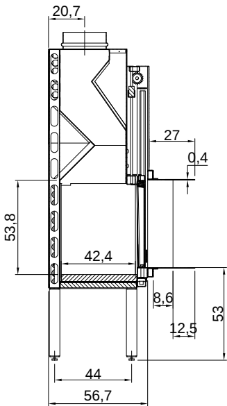
SEZIONE A-A
