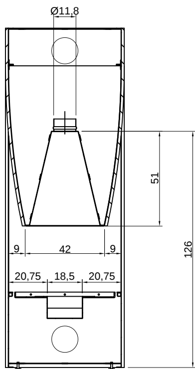
SEZIONE A-A
