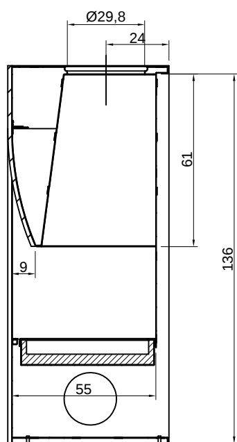
SEZIONE A-A
