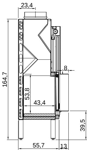
SEZIONE A-A
