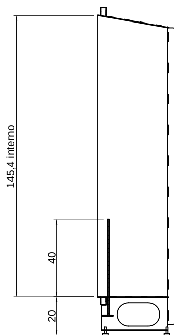
SEZIONE A-A
