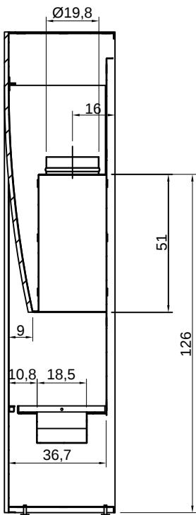
SEZIONE A-A
