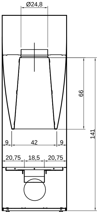
SEZIONE A-A
