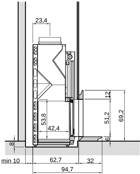
SEZIONE A-A
