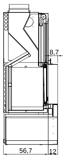
SEZIONE A-A
