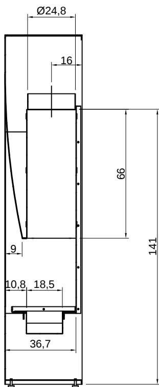
SEZIONE A-A
