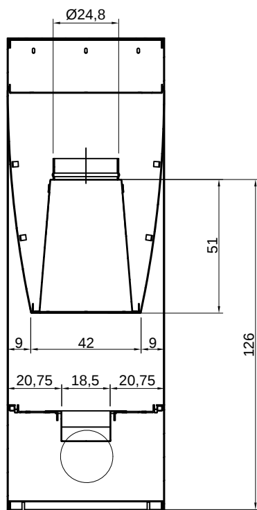
SEZIONE A-A
