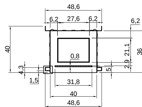
SEZIONE B-B
