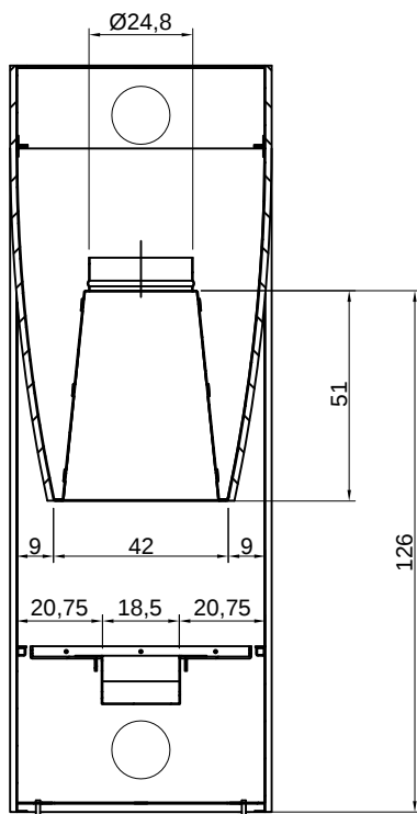
SEZIONE A-A
