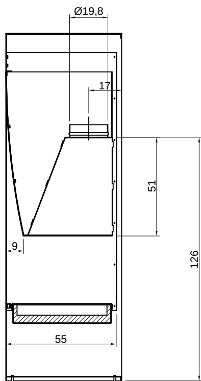
SEZIONE A-A
