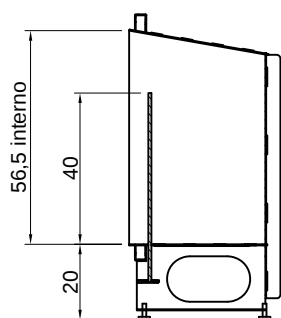
SEZIONE A-A
