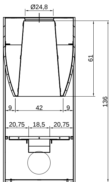
SEZIONE A-A
