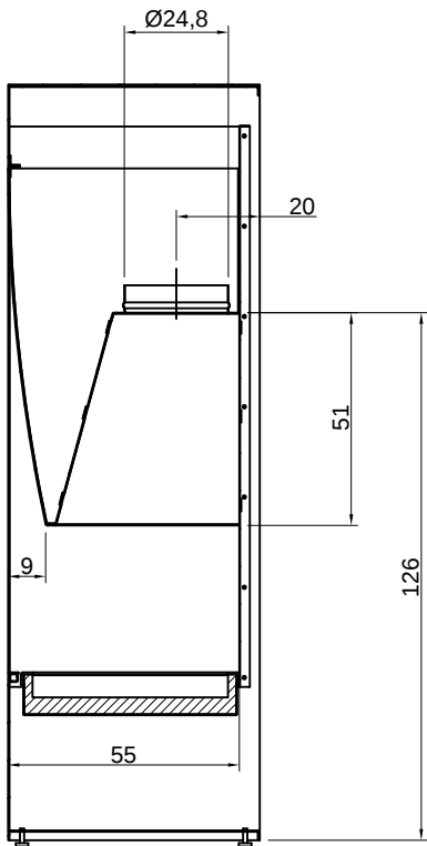
SEZIONE A-A
