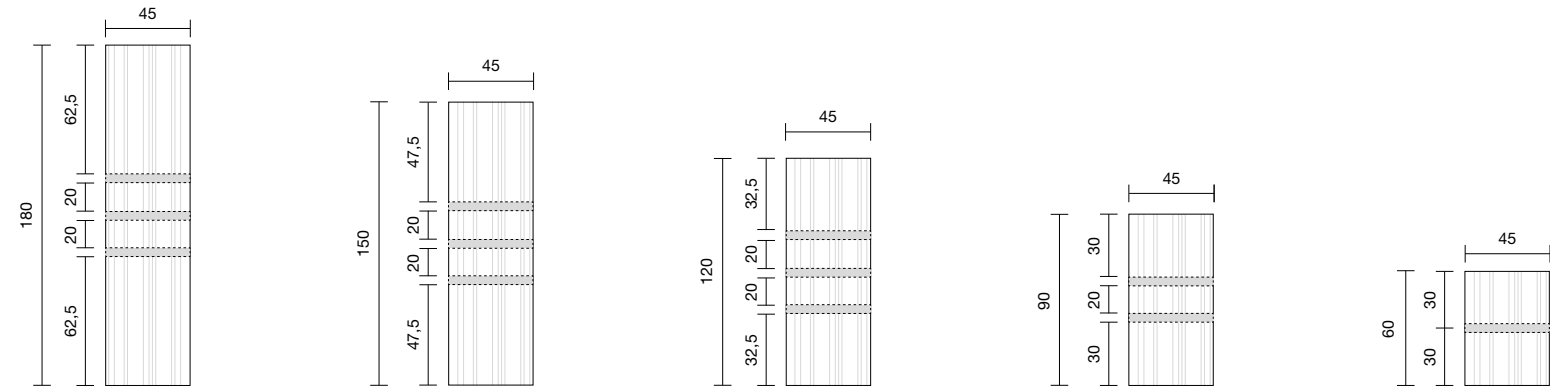
Possibile posizionamento per porta salviette Art. BITBARRA. Possible position of towel holder Art. BITBARRA.
