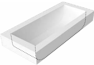
BIBLI080 H 53,5 P 80 L 180 cm BIBLI081 H 53,5 P 90 L 190 cm
