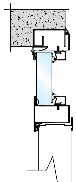
SEZIONE VERTICALE ANTA CON SOPRALUCE Vertical section of transom glass leaf Sección vertical hoja con lumbrera
