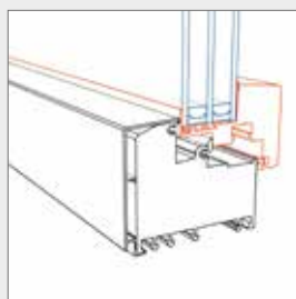
FIN-90 Nova-line N alluminio-PVC
