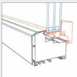
FIN-90 Nova-line C alluminio-PVC
