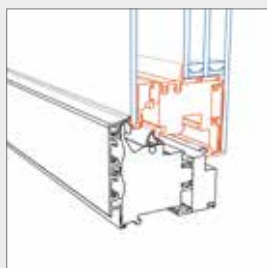
FIN-Project Nova-line Cristal Twin alluminio-alluminio, disponibile anche in legno e ForRes all'interno o senza anta accoppiata Twin
