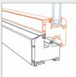
FIN-72 Step-line alluminio-PVC
