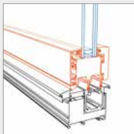
FIN-Fold Slim-line alluminio-legno, disponibile anche in alluminio all'interno
