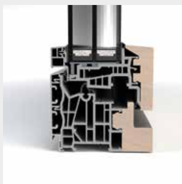
FIN-Project alluminio-legno
