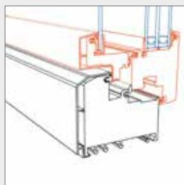
FIN-90 Classic-line Twin C alluminio-PVC, disponibile anche in PVC-PVC
