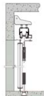
Posa oltre luce Installation to the wall Einbau auf der Wand
