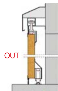
Appoggiato con ruote su guida Leaning with wheels on track Aufliegend, mit Bodenlaufrollen
