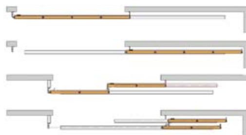
Configurazioni telescopiche Telescopic configurations Telescopische Darstellung
