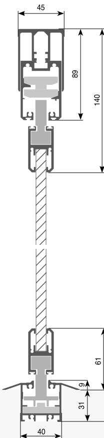
Sezione verticale guida incassata
