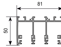
Guida superiore 3 binari
