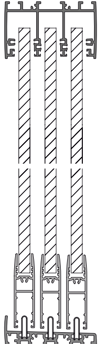
Sezione verticale
