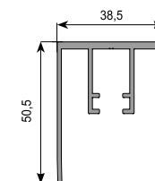
Profilo compensatore
