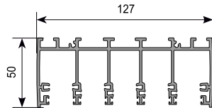
Guida superiore 5 binari
