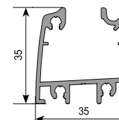
Guida inferiore
