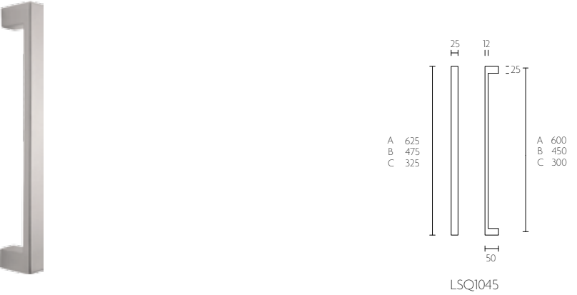
LSQ1045 massieve greep tbv houten, glazen of aluminium deuren doorgaande, niet-doorgaande of paarsgewijze bevestiging | solid pull handle for timber, glass or aluminium doors bolt-through, concealed or back to back fixings
