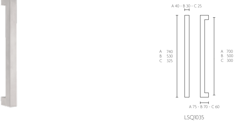
LSQ1035 massieve greep tbv houten, glazen of aluminium deuren doorgaande, niet-doorgaande of paarsgewijze bevestiging | solid pull handle for timber, glass or aluminium doors bolt-through, concealed or back to back fixings
