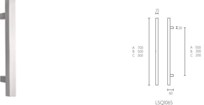
LSQ1065 massieve greep tbv houten, glazen of aluminium deuren doorgaande, niet-doorgaande of paarsgewijze bevestiging | solid pull handle for timber, glass or aluminium doors bolt-through, concealed or back to back fixings
