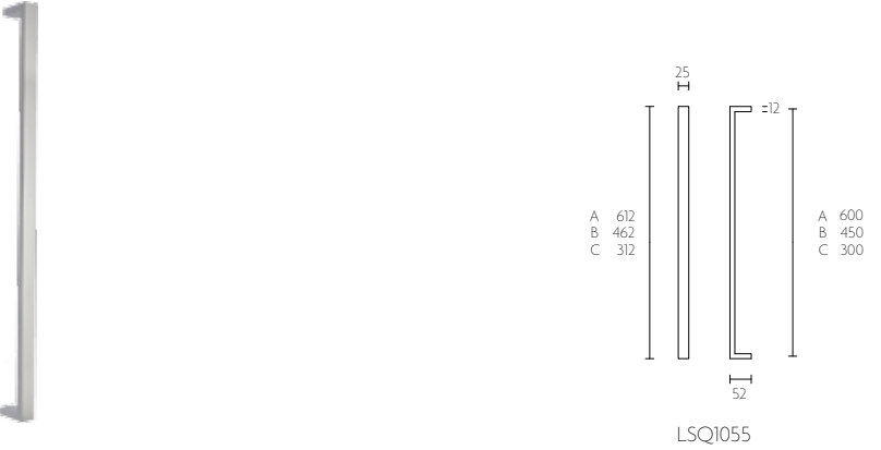
LSQ1055 massieve greep tbv houten, glazen of aluminium deuren doorgaande en paarsgewijze bevestiging | solid pull handle for timber, glass or aluminium doors bolt-through and back to back fixings
