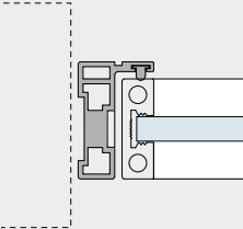
Muratura - Cartongesso Brickwall - Plasterboard
