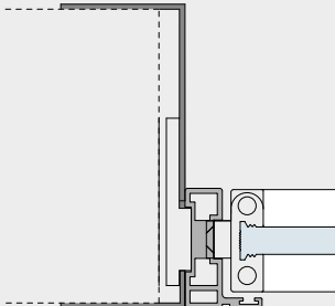
Muratura - Cartongesso Brickwall - Plasterboard
