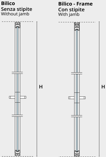
Altezze fino a 2700 mm Height up tp 2700 mm
