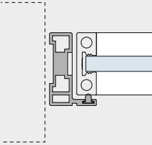
Muratura - Cartongesso Brickwall - Plasterboard
