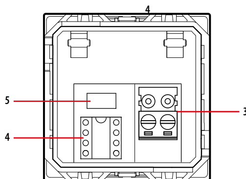
Vista posteriore
