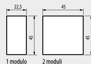
1 modulo
