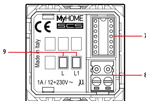
Vista posteriore
