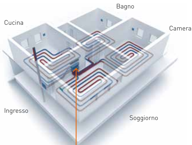
Esempio di impianto diviso a Zone con riscaldamento a pannelli radianti
