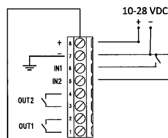
Vista dettagliata del connettore
