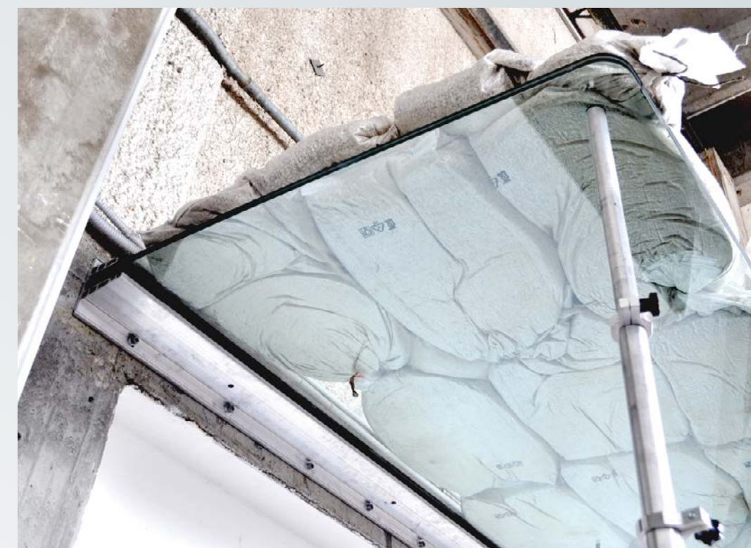
900 Kg TOTALI SU UNA PENSILINA DA 200 X 150 cm
