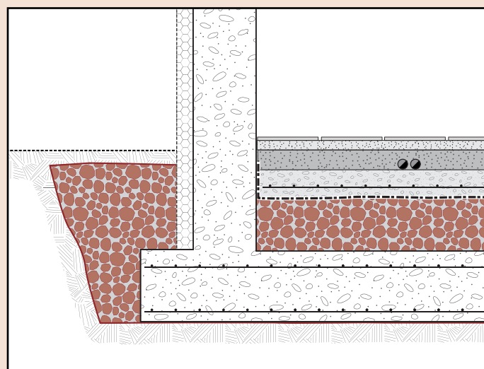
4 Isolamento sopra platea di fondazione. Sottofondo isolato in Leca TermoPiù sfuso/imboiaccato/cementato.
