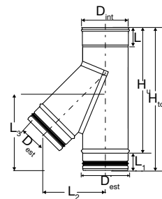
Dal Ø 300 al Ø 400 mm From Ø 300 to Ø 400 mm
