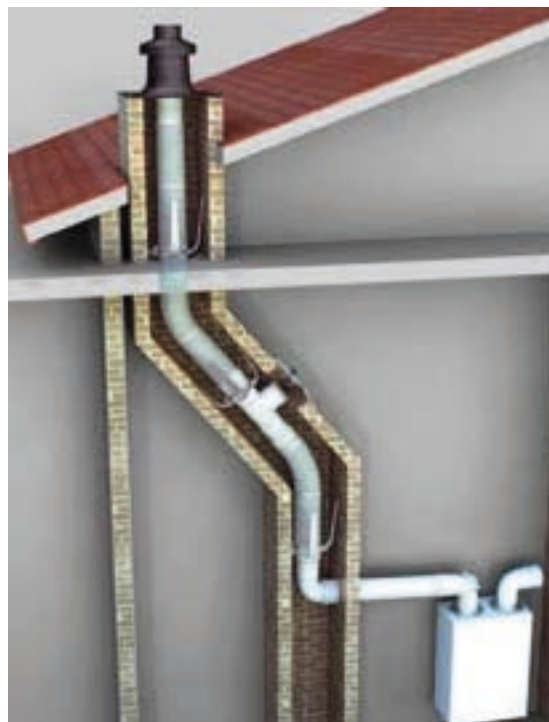
Sistema misto flex/rigido.
