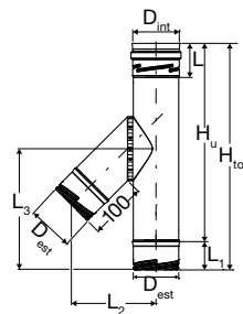
Dal Ø 80 al Ø 250 mm From Ø 80 to Ø 250 mm
