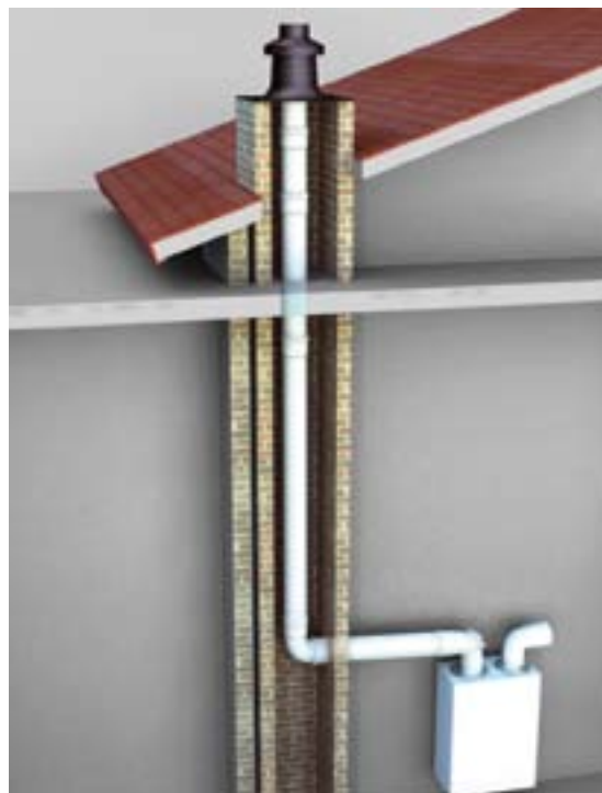
Sistema totalmente rigido.
