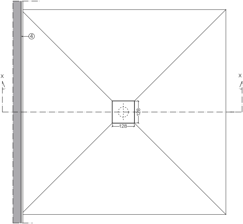
pianta piatto doccia - shower tray layout
