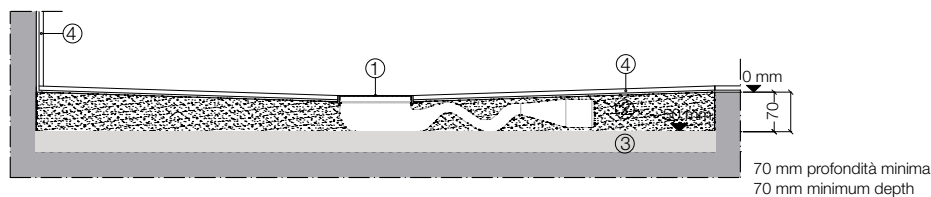
sez. X-X piatto doccia - section X-X shower tray
