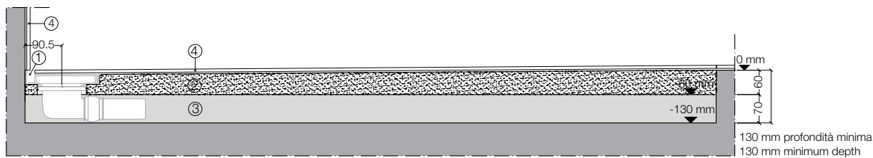
sez. X-X piatto doccia - section X-X shower tray
