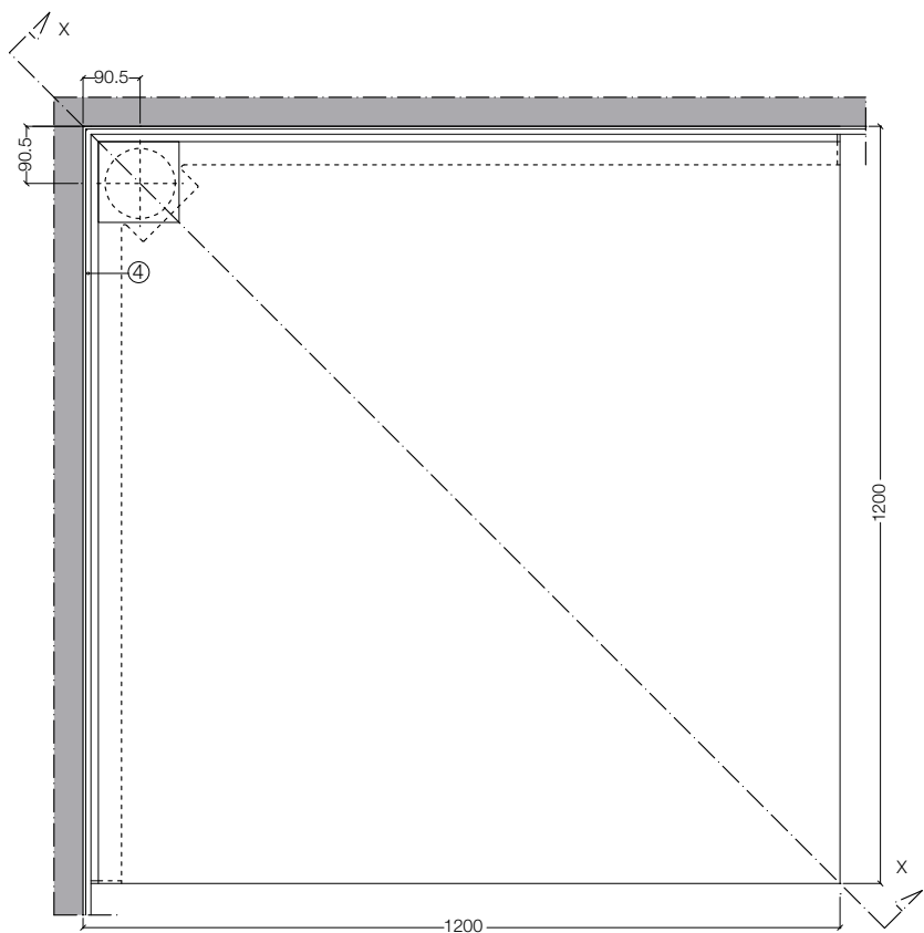
pianta piatto doccia - shower tray layout
