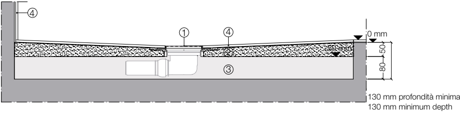
sez. X-X piatto doccia - section X-X shower tray
