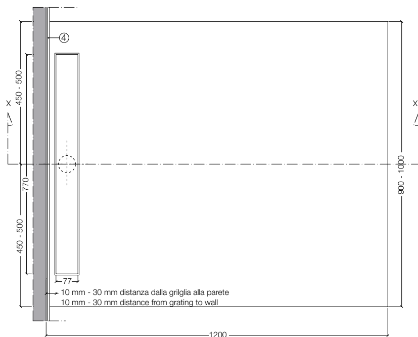
pianta piatto doccia - shower tray layout
