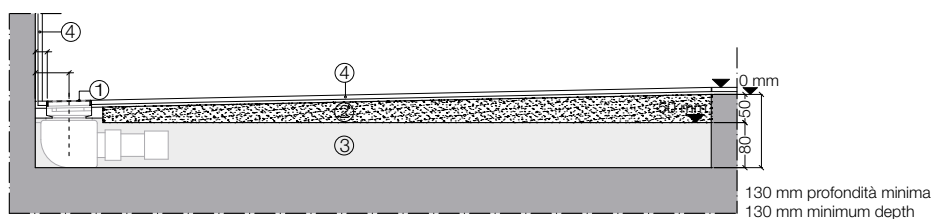
sez. X-X piatto doccia - section X-X shower tray
