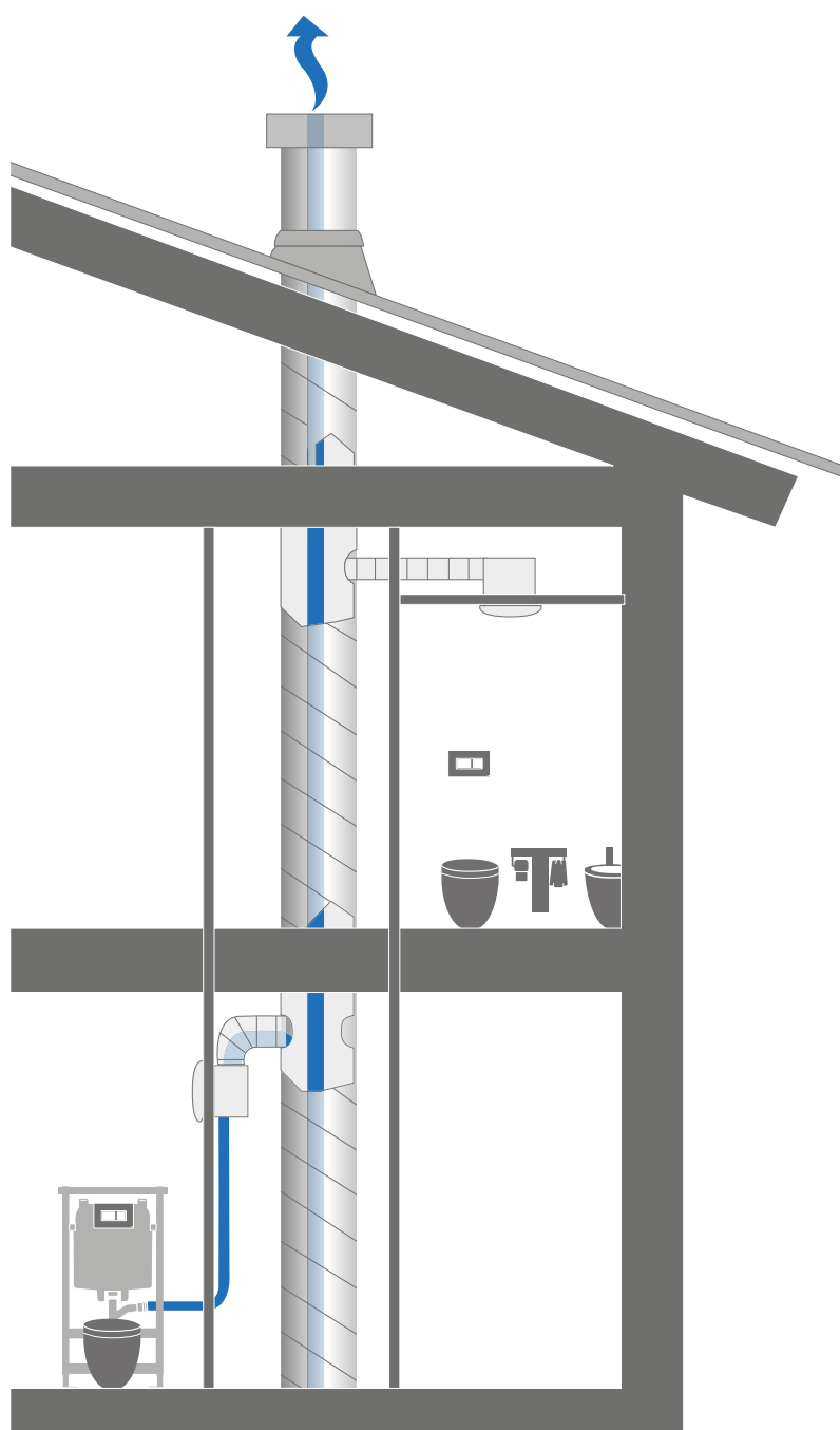
Uscita su colonna di ventilazione
