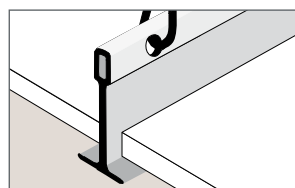
Pannelli con bordo A per struttura a vista
