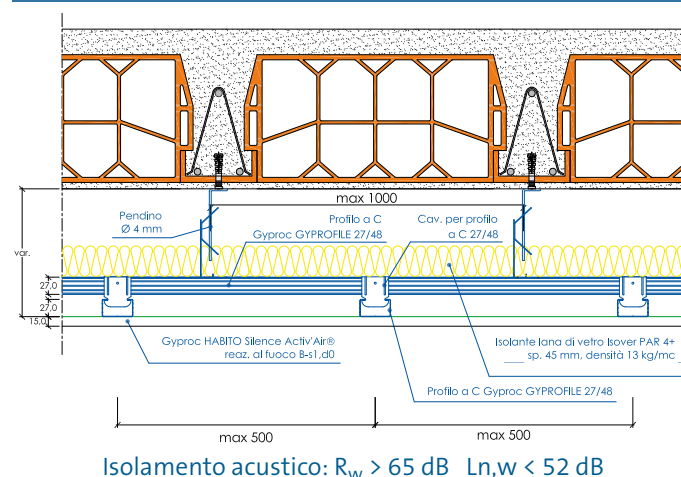
Controsoffitto continuo Gyproc CS.ACU L Habito Silence Activ'Air®
