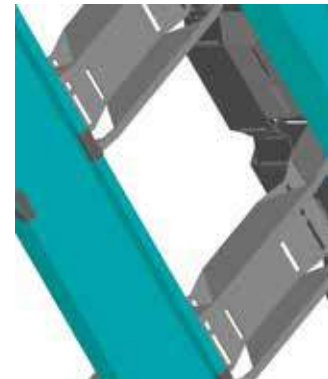
Dettaglio raccordo
