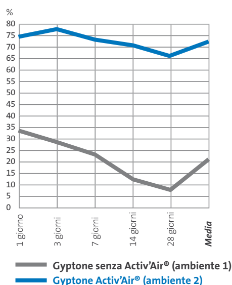
Riduzione della formaldeide dopo 3 mesi (%)
