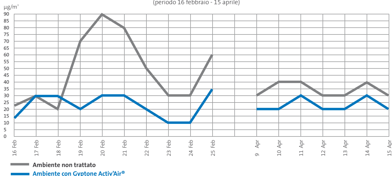
Concentrazione della formaldeide nell'aria (periodo 16 febbraio - 15 aprile)
