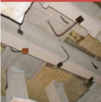
Elementi prima della prova al fuoco
