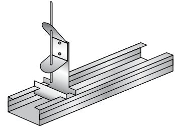
Dettaglio raccordo
