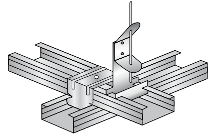
Dettaglio raccordo
