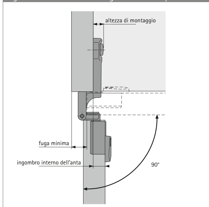
Ingombro interno dell'anta e fuga minima con apertura a 90°
