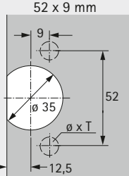
Schema di foratura 52 x 9 mm
