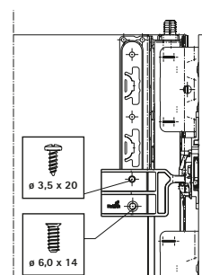
Trascinatore montato
