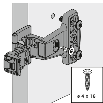
Con bussole a espansione premontate
