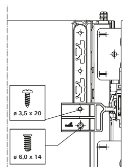
Trascinatore montato
