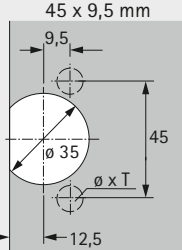
Schema di foratura 45 x 9,5 mm
