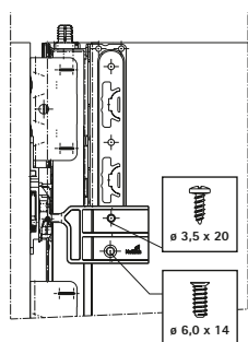
Trascinatore montato
