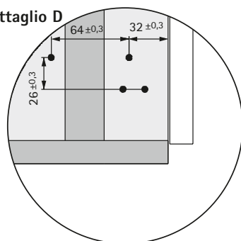
Sezione C-C
