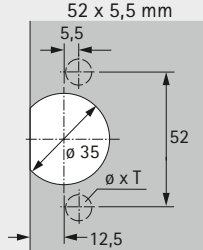
Schema di foratura 52 x 5,5 mm
