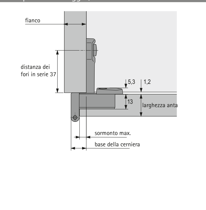
Esempio di montaggio, anta chiusa
