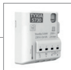
TYXIA 5730 Delta Dore Ricevitore radio collegabile via cavo ad un relé di commutazione da incasso di ogni tipo e marca 12/24 V da collegare alla centralina Tronic
