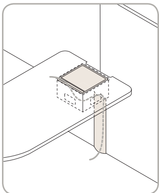
en_Flap and fabric cable riser, for meeting table it_Sportello e calza per salita cavi, per tavolo riunione fr_Top access et chemin de câbles, pour table de réunion
