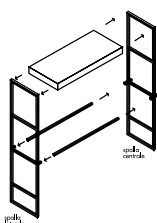
esemplificazione montaggio
