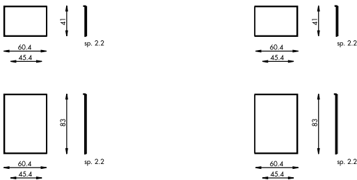
esemplificazione montaggio
