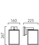
BOX LANTERN 270
