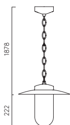
PORTREE PENDANT
