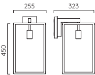
BOX LANTERN 450
