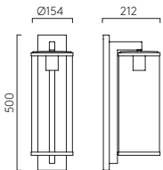
PIMLICO 500
