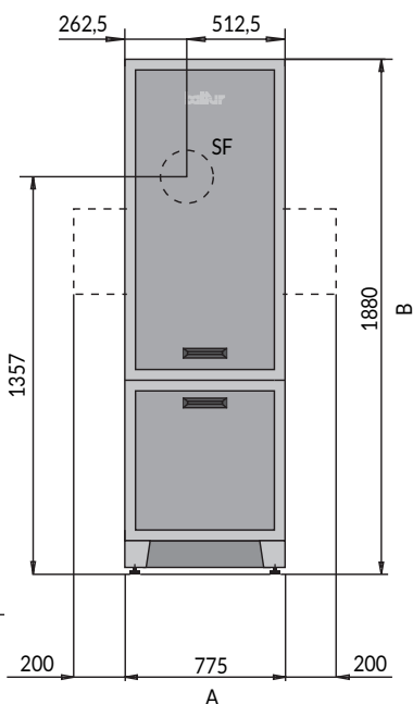
VISTA FRONTALE
