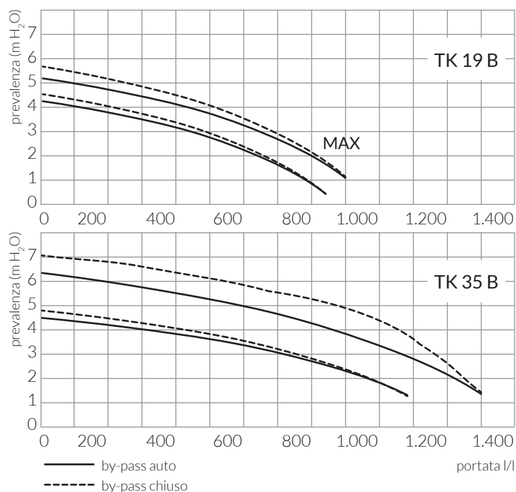
DIAGRAMMA PORTATA-PREVALENZA DISPONIBILE ALL'IMPIANTO
