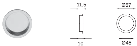
2193 rosetta incasso sliding door handle
