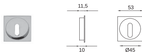
2185/F rosetta incasso foro chiave sliding door handle key hole
