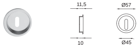
2193/F rosetta incasso foro chiave sliding door handle key hole
