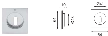
SD221 rosetta incasso foro chiave sliding door handle key hole
