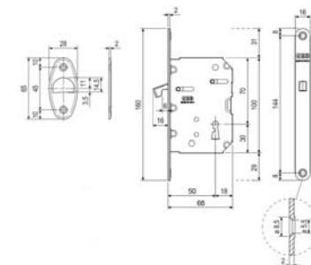
SD205 set rosette incasso foro chiave con frontale + serratura sliding door handle set key hole with flush pull hole + lock
