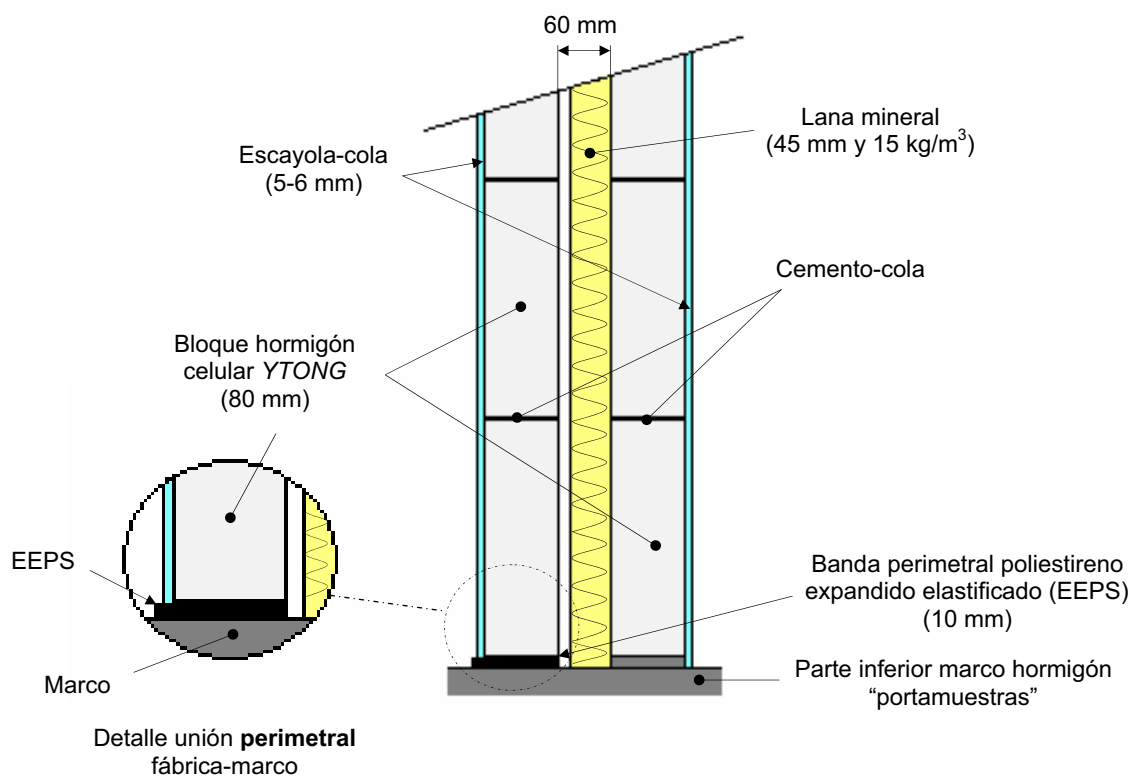
Figura 1: Esquema de muestra ensayada (B1001-9-M1)
