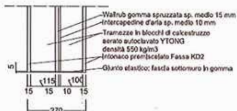
Particolare B
