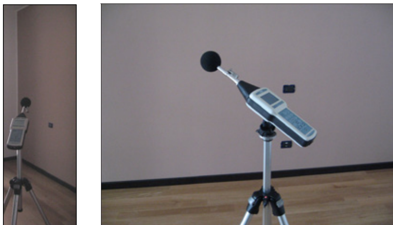
Fig. 4 – Partizione misurata – foto dall'interno
