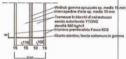
Particolare B
