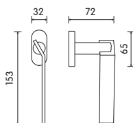
MP 2020 FR5 Maniglia finestra con movimento 4 scatti Window handle with 4 clicks position
