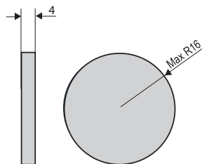
Dima per foro Hole template
