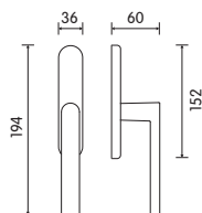
MP 2013 BC F Maniglia finestra su placca Window handle on plate
