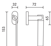
MP 2020 BC FR5 Maniglia finestra con movimento 4 scatti Window handle with 4 clicks position
