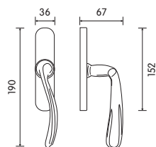
MP 3006 F Maniglia finestra su placca Window handle on plate
