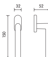
MP 2013 BC FR5 Maniglia finestra con movimento 4 scatti Window handle with 4 clicks position
