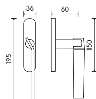
MP 2020 F Maniglia finestra su placca Window handle on plate
