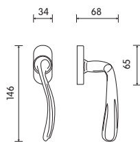
MP 3006 FR5 Maniglia finestra con movimento 4 scatti Window handle with 4 clicks position
