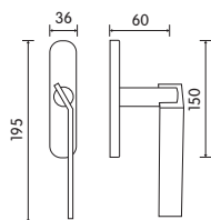
MP 2020 BC F Maniglia finestra su placca Window handle on plate
