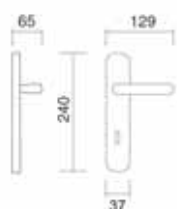
Art. 3300 Maniglia su placca Handle on plate
