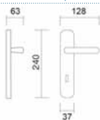
Art. 3390 Maniglia su placca Handle on plate
