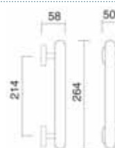
Art. 2865 Maniglione Pull handle
