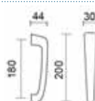
Art. 0117/ Maniglione su placca Pull Handle on plate
