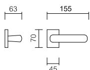
Art. 3921/3421 Maniglia su rosetta Handle on rose
