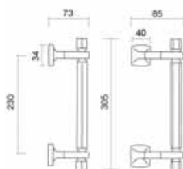
Art. 0105 Maniglione Esagonale Pull handle Esagonale
