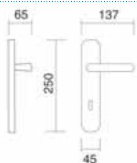
Art. 3100 Maniglia su placca Handle on plate
