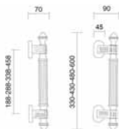
Art. 0220 Maniglione Impero Pull handle Impero
