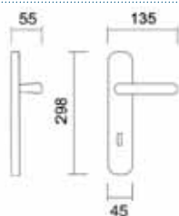
Art. 3770/3740 Maniglia su placca Handle on plate
