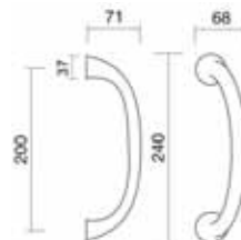
Art. 3255 Maniglione Giza Pull handle Giza
