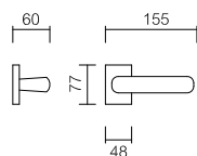
Art. 8261 Maniglia su rosetta originale Handle on rose
