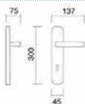
Art. 3740 Maniglia su placca Handle on plate
