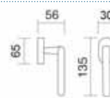
Art. 2798 Dreh kipp Dreh kipp
