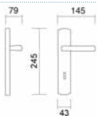
Art. 3050 Maniglia su placca Handle on plate
