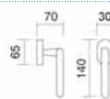
Art. 2808 Dreh kipp Dreh kipp
