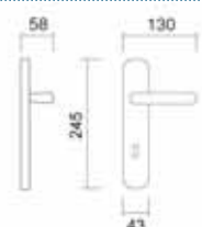
Art. 3470 Maniglia su placca Handle on plate
