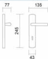
Art. 3250 Maniglia su placca Handle on plate
