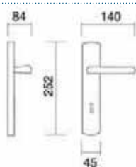
Art. 3210 Maniglia su placca Handle on plate
