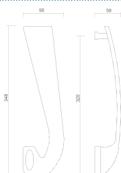
Art. 0118/C Maniglione Rimira Pull handle Rimira
