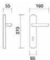
Art. 3720 Maniglia su placca Handle on plate
