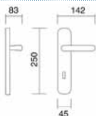
Art. 2840 Maniglia su placca Handle on plate
