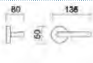
Art. 2781 Maniglia su rosetta Handle on rose
