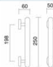
Art. 3085 Maniglione Pull handle
