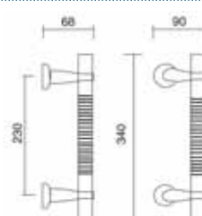
Art. 0412/AI Maniglione Royal righe Pull handle Royal righe
