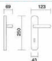
Art. 2970 Maniglia su placca Handle on plate
