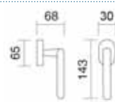
Art. 3108 Dreh kipp Dreh kipp
