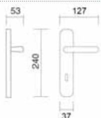
Art. 2790 Maniglia su placca Handle on plate
