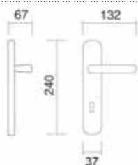
Art. 2800 Maniglia su placca Handle on plate
