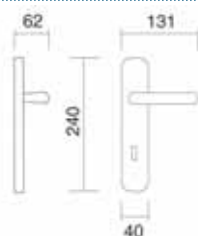
Art. 0020 Maniglia su placca Handle on plate
