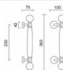
Art. 0107/R Maniglione Giava Pull handle Giava
