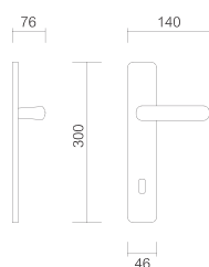
Art. 2016/3740 Maniglia su placca Handle on plate
