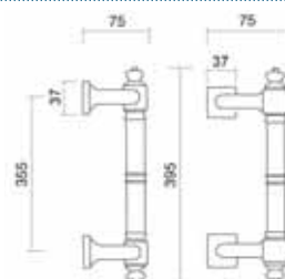
Art. L652-2 Maniglione Creta doppio Pull handle Creta doppio
