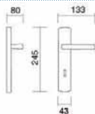
Art. 2780 Maniglia su placca Handle on plate
