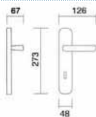
Art. 2960 Maniglia su placca Handle on plate
