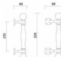
Art. 0107/AI Maniglione Giava Pull handle Giava
