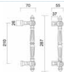
Art. 0550 Maniglione Patrizio Pull handle Patrizio
