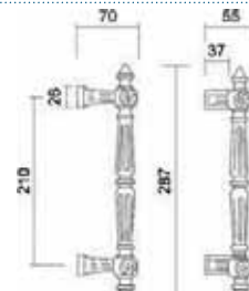
Art. 0550 Maniglione Pull handle
