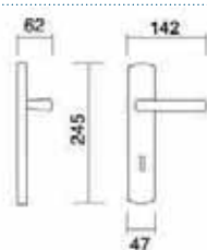
Art. 3230 Maniglia su placca Handle on plate
