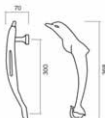
Art. 0420 Maniglione Pull handle
