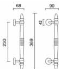
Art. 0410/AI Maniglione Royal stile Pull handle Royal stile
