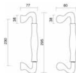
Art. 0244 Maniglione Zodiaco Acquarius g.spostato Pull handle Zodiaco Acquarius g.spostato
