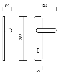
Art. 8260 Maniglia su placca Handle on plate
