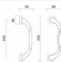
Art. 3155 Maniglione Lybra Pull handle Lybra
