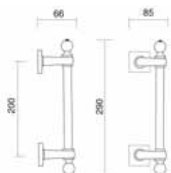
Art. 0656 Maniglione Creta gambo tondo p/b Pull handle Creta round foot p/b
