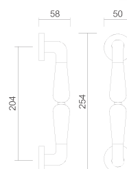
Art. 3515 Maniglione Pull handle
