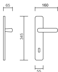
Art. 3920 Maniglia su placca Handle on plate
