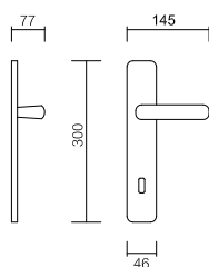
Art. 3820 Maniglia su placca Handle on plate
