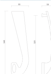
Art. 0118 Maniglione Rimira Pull handle Rimira
