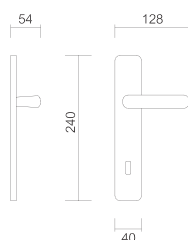
Art. 3650 Maniglia su placca Handle on plate
