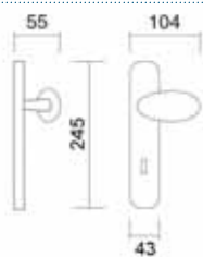
Art. 3580 Maniglia su placca Handle on plate
