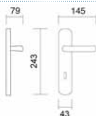
Art. 3060/3520 Maniglia su placca Handle on plate
