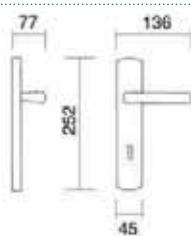
Art. 3220 Maniglia su placca Handle on plate
