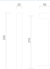
Art. 3865 Maniglione Pull Handle
