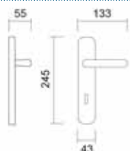
Art. 3380 Maniglia su placca Handle on plate
