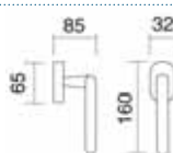
Art. 3758 Dreh kipp Dreh kipp
