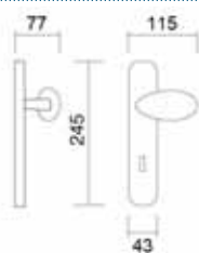
Art. 3170 Maniglia su placca Handle on plate
