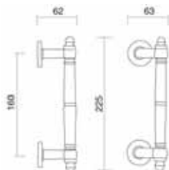
Art. 0034 Maniglione Zancato Pull handle Zancato
