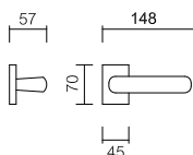
Art. 3811/3421 Maniglia su rosetta Handle on rose
