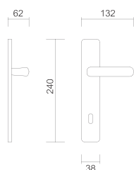
Art. 3850 Maniglia su placca Handle on plate
