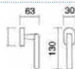
Art. 1808 Dreh kipp Dreh kipp
