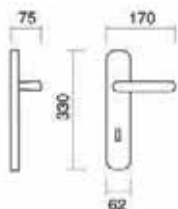
Art. 3660 Maniglia su placca Handle on plate
