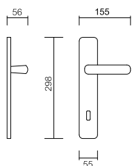
Art. 3810 Maniglia su placca Handle on plate
