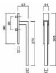
Art. 3547 Maniglione Anta ribalta quadrato Pull handle Anta ribalta quadrato
