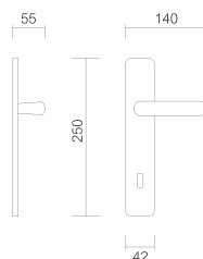
Art. 3860 Maniglia su placca Handle on plate
