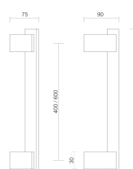
Art. 3035 Maniglione Phoenix Pull handle Phoenix
