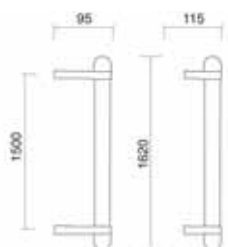
Art. 3027 Maniglione Spazio Pull handle Spazio
