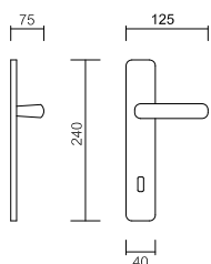
Art. 8270 Maniglia su placca Handle on plate
