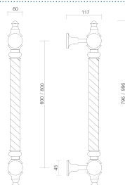
Art. 0119 Maniglione Scettro Pull handle Scettro
