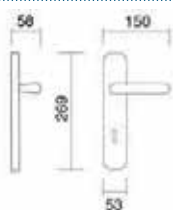
Art. 3360 Maniglia su placca Handle on plate
