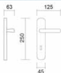
Art. 1010 Maniglia su placca Handle on plate
