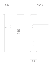
Art. 3840 Maniglia su placca Handle on plate
