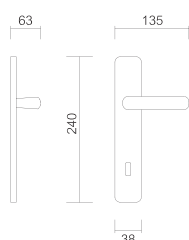
Art. 3510 Maniglia su placca Handle on plate
