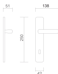
Art. 3760/ Maniglia su placca Handle on plate
