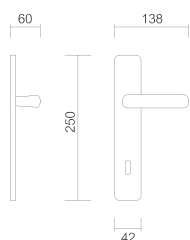
Art. 3830 Maniglia su placca Handle on plate
