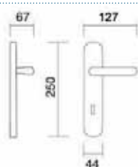
Art. 1440 Maniglia su placca Handle on plate
