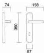
Art. 3780 Maniglia su placca Handle on plate
