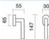
Art. 0038 Dreh kipp Dreh kipp
