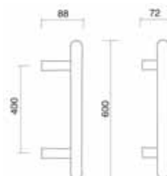
Art. 3028 Maniglione Galassia Pull handle Galassia
