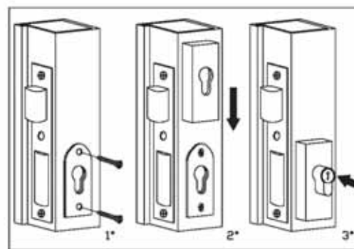
ISTRUZIONI MONTAGGIO BOCCHETTE SICUREZZA
