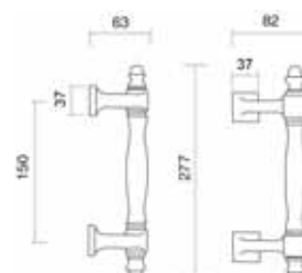
Art. 0653 Maniglione Cipro Pull handle Cipro
