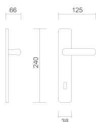
Art. 3270 Maniglia su placca Handle on plate
