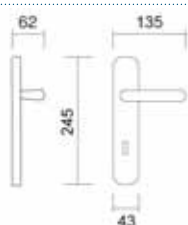
Art. 3320 Maniglia su placca Handle on plate
