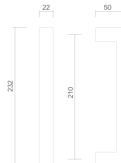
Art. 3875 Maniglione Pull Handle
