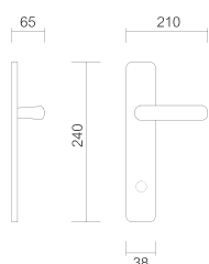
Art. 8310 Maniglia su placca Handle on plate
