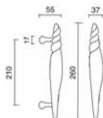
Art. 0114 Maniglione Conchiglia Pull handle Conchiglia
