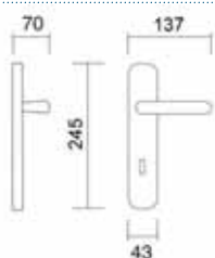
Art. 3480 Maniglia su placca Handle on plate
