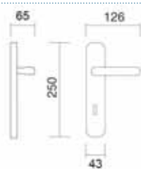
Art. 2950 Maniglia su placca Handle on plate
