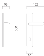
Art. 7100 Maniglia su placca Handle on plate
