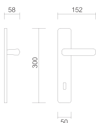
Art. 7100 Maniglia su placca Handle on plate
