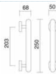
Art. 3075 Maniglione Pull handle
