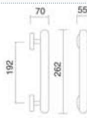
Art. 1335 Maniglione Pull handle
