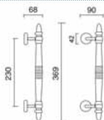
Art. 0410 Maniglione Royal stile Pull handle Royal stile
