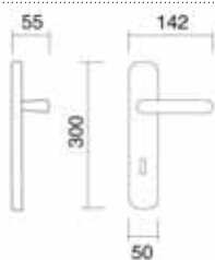
Art. 3540 Maniglia su placca Handle on plate
