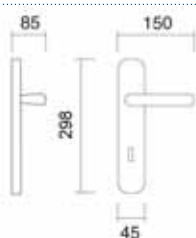
Art. 3750 Maniglia su placca Handle on plate
