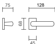
Art. 8271 Maniglia su rosetta Handle on rose
