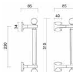
Art. 0106 Maniglione Semitondo Pull handle Semitondo
