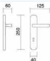
Art. 0030 Maniglia su placca Handle on plate
