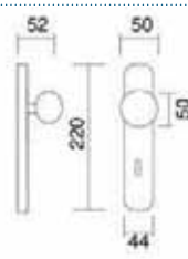
Art. 1446 Pomolo su placca Knob on plate
