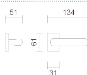
Art. 3771/0071 Maniglia su rosetta Handle on rose
