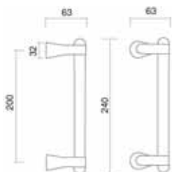
Art. 0441 Maniglione Zeta Pull handle Zeta
