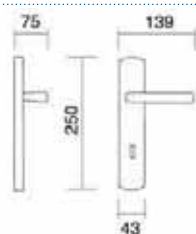
Art. 3150 Maniglia su placca Handle on plate
