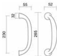
Art. 0315 Maniglione Trend Pull handle Trend
