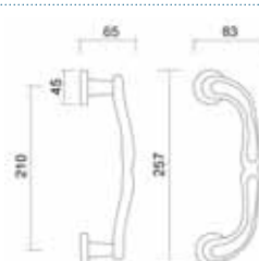
Art. 0069 Maniglione Sorriso Pull handle Sorriso
