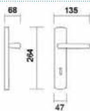
Art. 3420 Maniglia su placca Handle on plate
