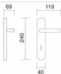
Art. 1330 Maniglia su placca Handle on plate
