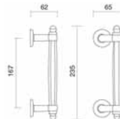
Art. 0175 Maniglione Ducale Pull handle Ducale
