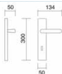
Art. 3670/3540 Maniglia su placca Handle on plate
