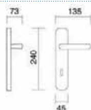
Art. 2830 Maniglia su placca Handle on plate
