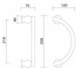
Art. 0111 Maniglione Luna Pull handle Luna
