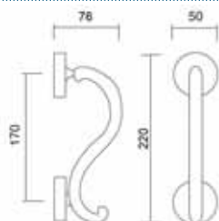
Art. 4020 Maniglione Vela Pull handle Vela
