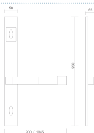
Art. 0121 Maniglione Misurati Pull handle Misurati
