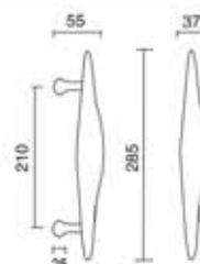
Art. 0115 Maniglione Corallo Pull handle Corallo
