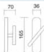
Art. 2868 Dreh kipp Dreh kipp
