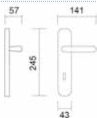
Art. 2860 Maniglia su placca Handle on plate
