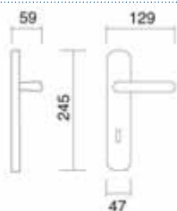
Art. 3080 Maniglia su placca Handle on plate
