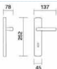
Art. 3200 Maniglia su placca Handle on plate
