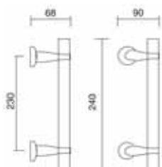
Art. 0411/AI Maniglione Royal liscio Pull handle Royal liscio
