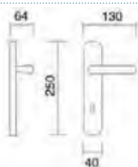
Art. 0300 Maniglia su placca Handle on plate
