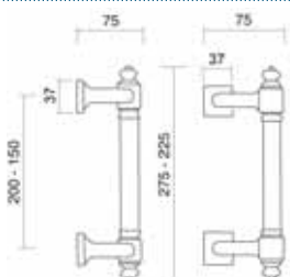
Art. L652 Maniglione Creta Pull handle Creta
