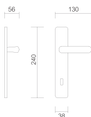
Art. 3880 Maniglia su placca Handle on plate
