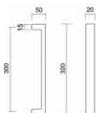
Art. M2602 Maniglione Arona Pull handle Arona
