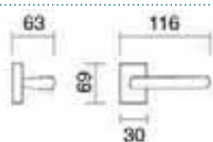
Art. 1801 Maniglia su rosetta Handle on rose
