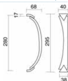
Art. 0112 Maniglione Olimpo Pull handle Olimpo
