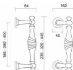
Art. 0211 Maniglione Pireo Medio Pull handle Pireo Medio
