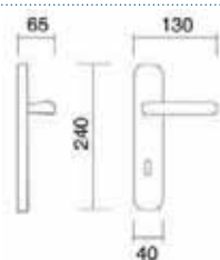
Art. 1050 Maniglia su placca Handle on plate
