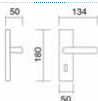
Art. 3670 Maniglia su placca corta Handle on plate
