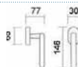
Art. 3228 Dreh kipp Dreh kipp
