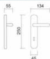
Art. 3280 Maniglia su placca Handle on plate
