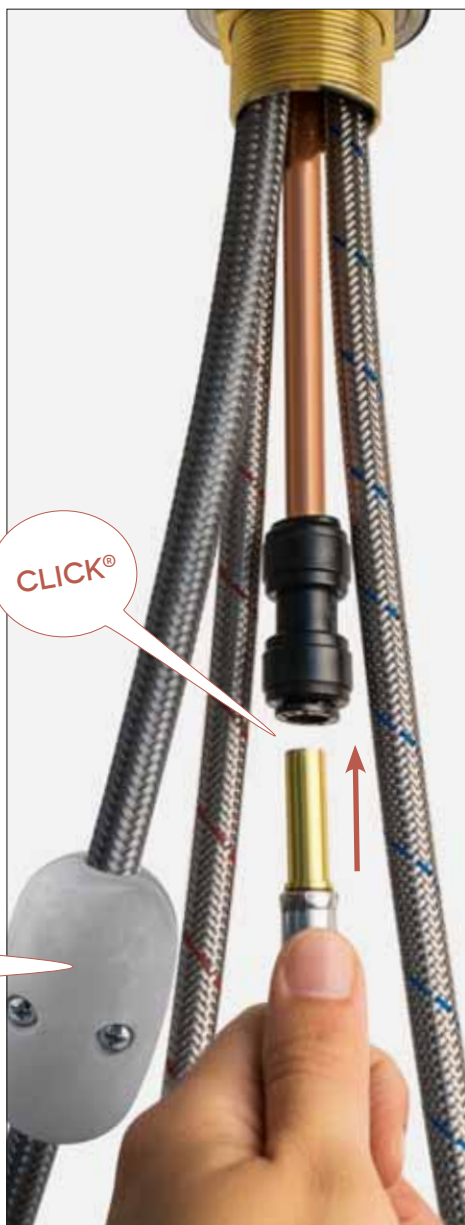
AGGANCIO RAPIDO E GARANTITO PER DOCCETTA ESTRAIBILE – Quick and secure connection for extractible handshower
