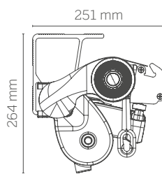
Modello ribassato
