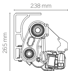
Modello classico
